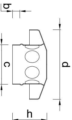
Doorsnede
