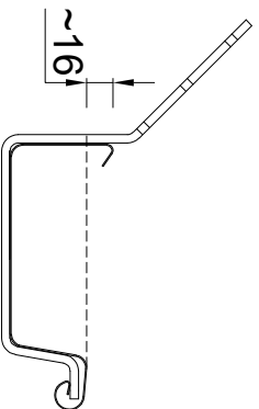
Goot B30 en beugel B30 Schaal 1:5
