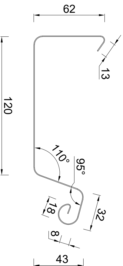
Doorsnede Schaal 1:2
