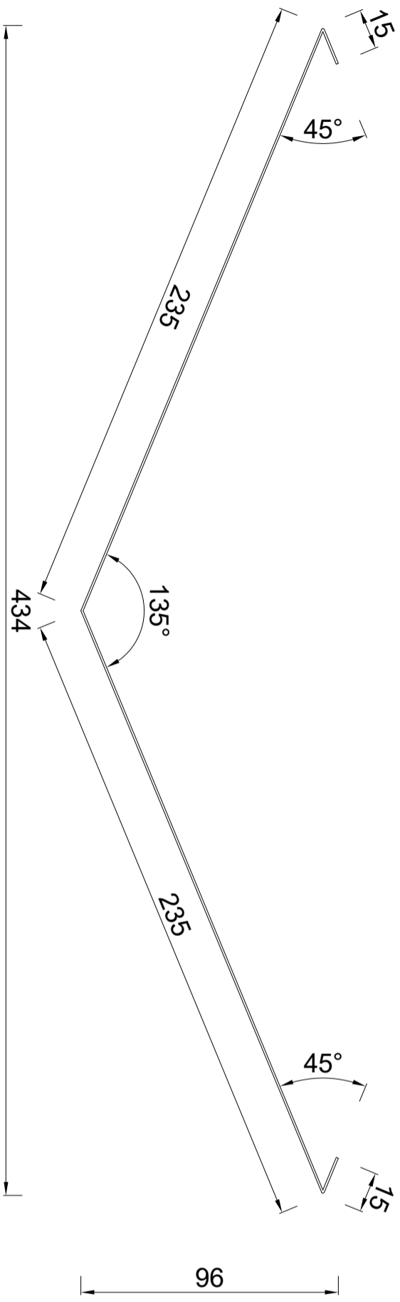
Doorsnede. Schaal 1:2
