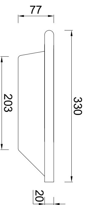
Zijaanzicht rechts
