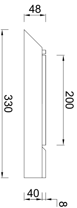
Bovenaanzicht rechts
