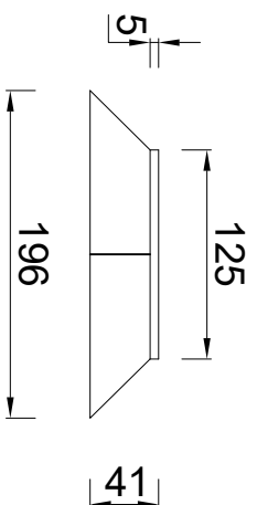
Bovenaanzicht
