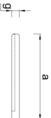
Bovenaanzicht rechts
