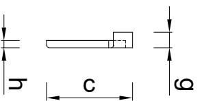
Vooraanzicht links
