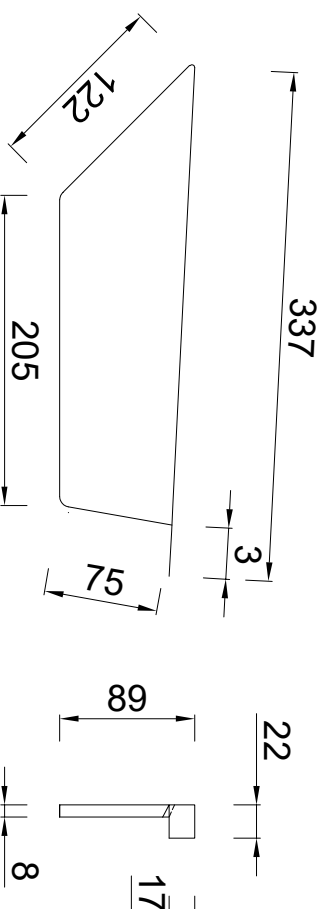
Zijanzicht rechts Vooranzicht rechts
