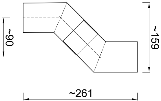
Doorsnede sprong
