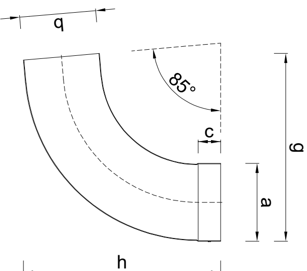
Doorsnede
