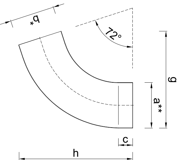
Doorsnede
