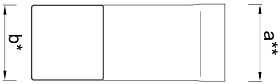
Voorraanzicht
