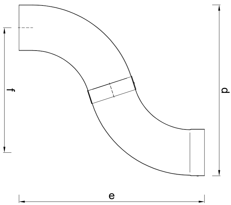
Doorsnede sprong
