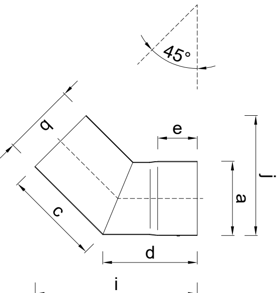
Doorsnede
