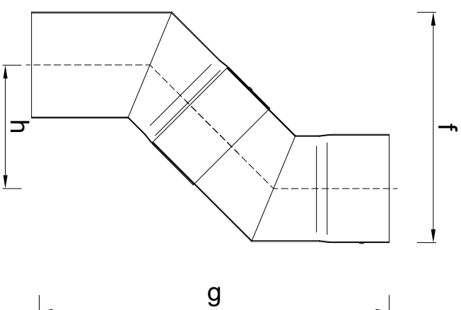
Doorsnede sprong
