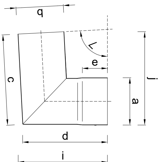
Doorsnede
