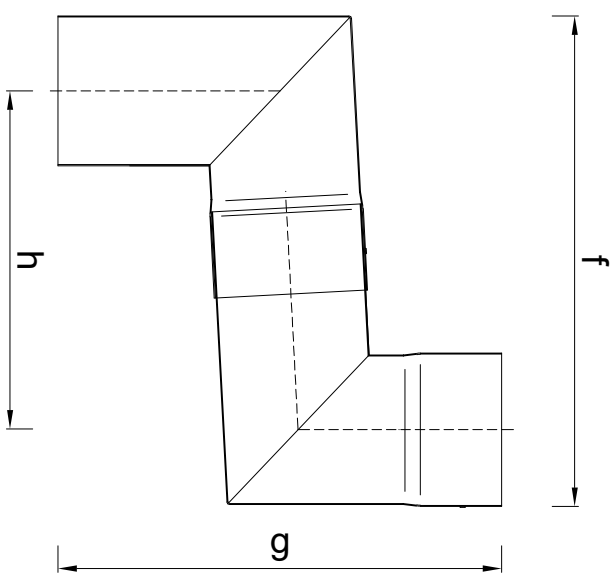
Doorsnede sprong
