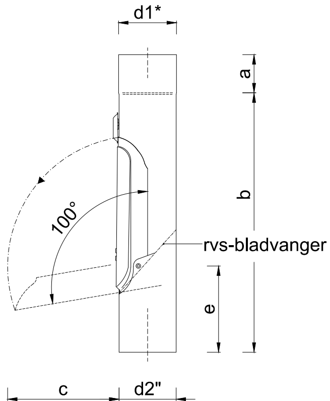
Zijaanzicht
