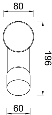
Bovenaanzicht
