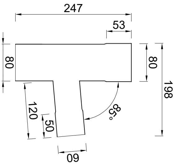
Doorsnede
