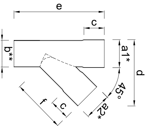
Doorsnede
