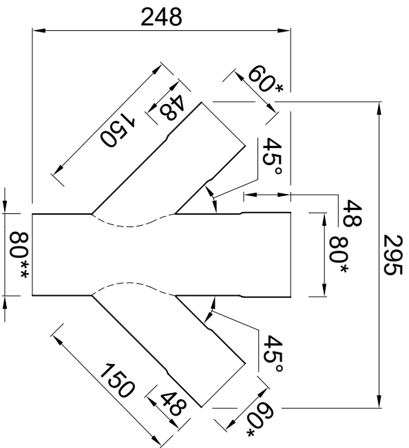
Doorsnede
