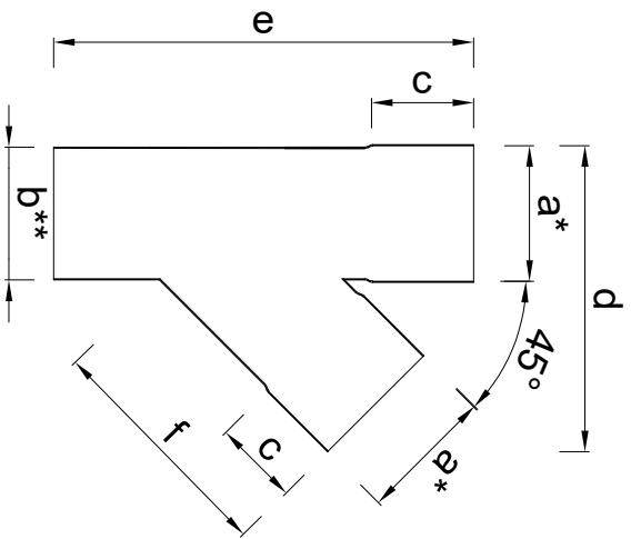
Doorsnede
