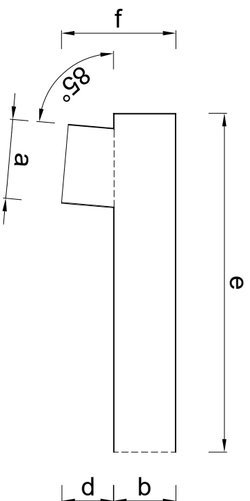
Doorsnede
