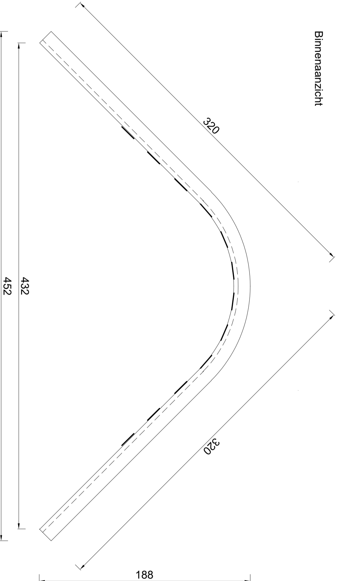
Bovenaanzicht
