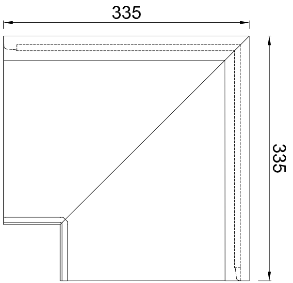
Zijaanzicht Rechts
