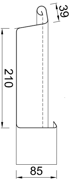
Doorsnede
