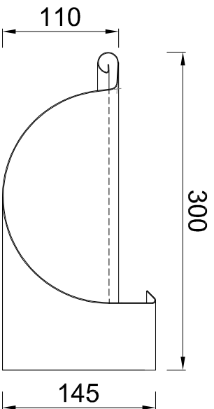
Doorsnede
