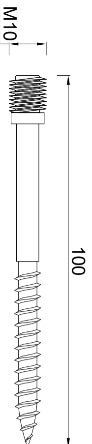
RHEINZINK schroefstift RVS voor scharnierpijpeugel M10x 100mm Artikelnummer: 2840001066
