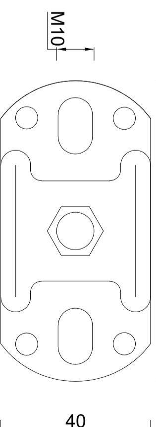
RHEINZINK gegalvaniseerde montageplaat M10 t.b.v. scharnierpijpeugel Artikelnummer: 2840001410
