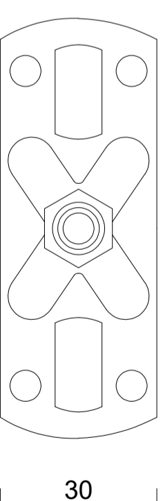
RHEINZINK rvs montageplaat M8/M10 t.b.v. scharnierpijpeugel Artikelnummer: 2840001414
