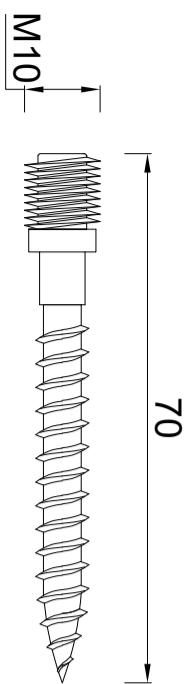
RHEINZINK schroefstift RVS voor scharnierpijpeugel M10x 70mm Artikelnummer: 2840001065
