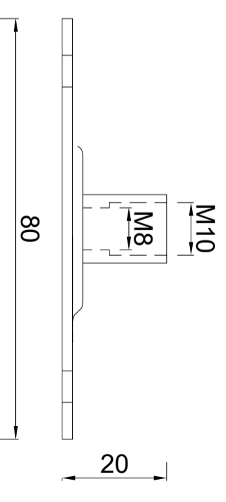
RHEINZINK gegalvaniseerde montageplaat M10 t.b.v. scharnierpijpeugel Artikelnummer: 2840001410
