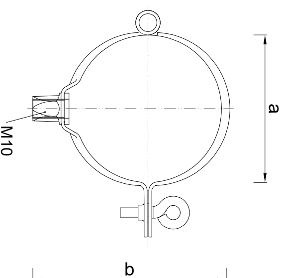
Bovenaanzicht
