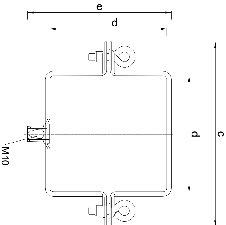
Bovenaanzicht
