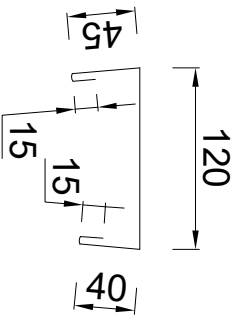
Gootbladvanger Doorsnede. Schaal 1:5
