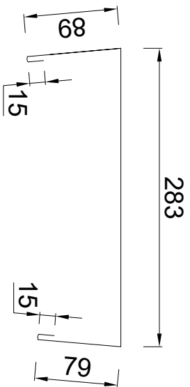
Gootbladvanger Doorsnede: Schaal 1:5
