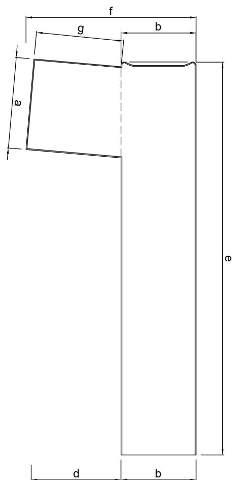
Doorsnede
