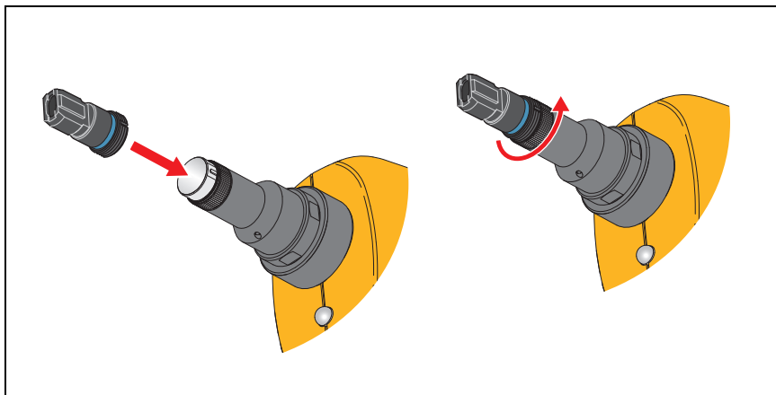
Figura 43. Conexión de punta MPO
