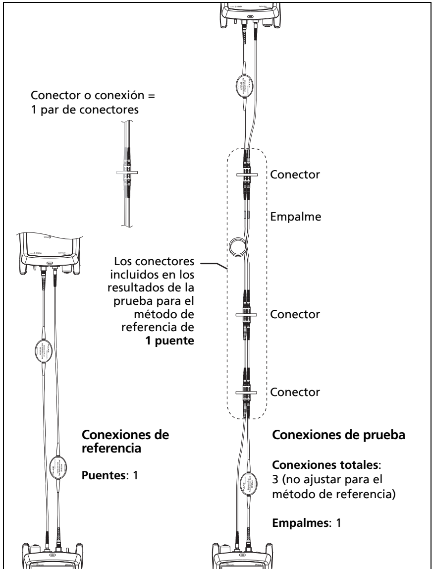
Figura 59. Cómo contar el número de conectores, empalmes y puentes
