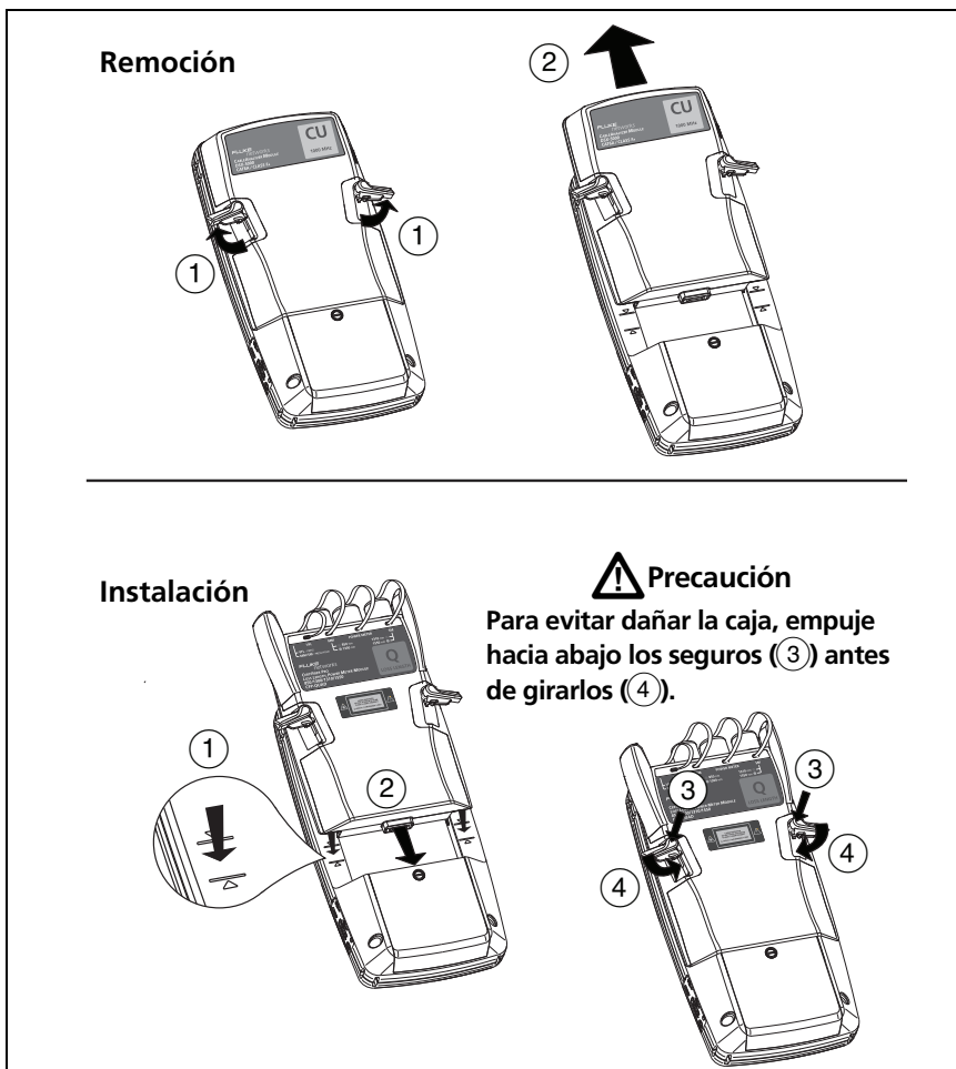
Figura 6. Cómo quitar e instalar un módulo
