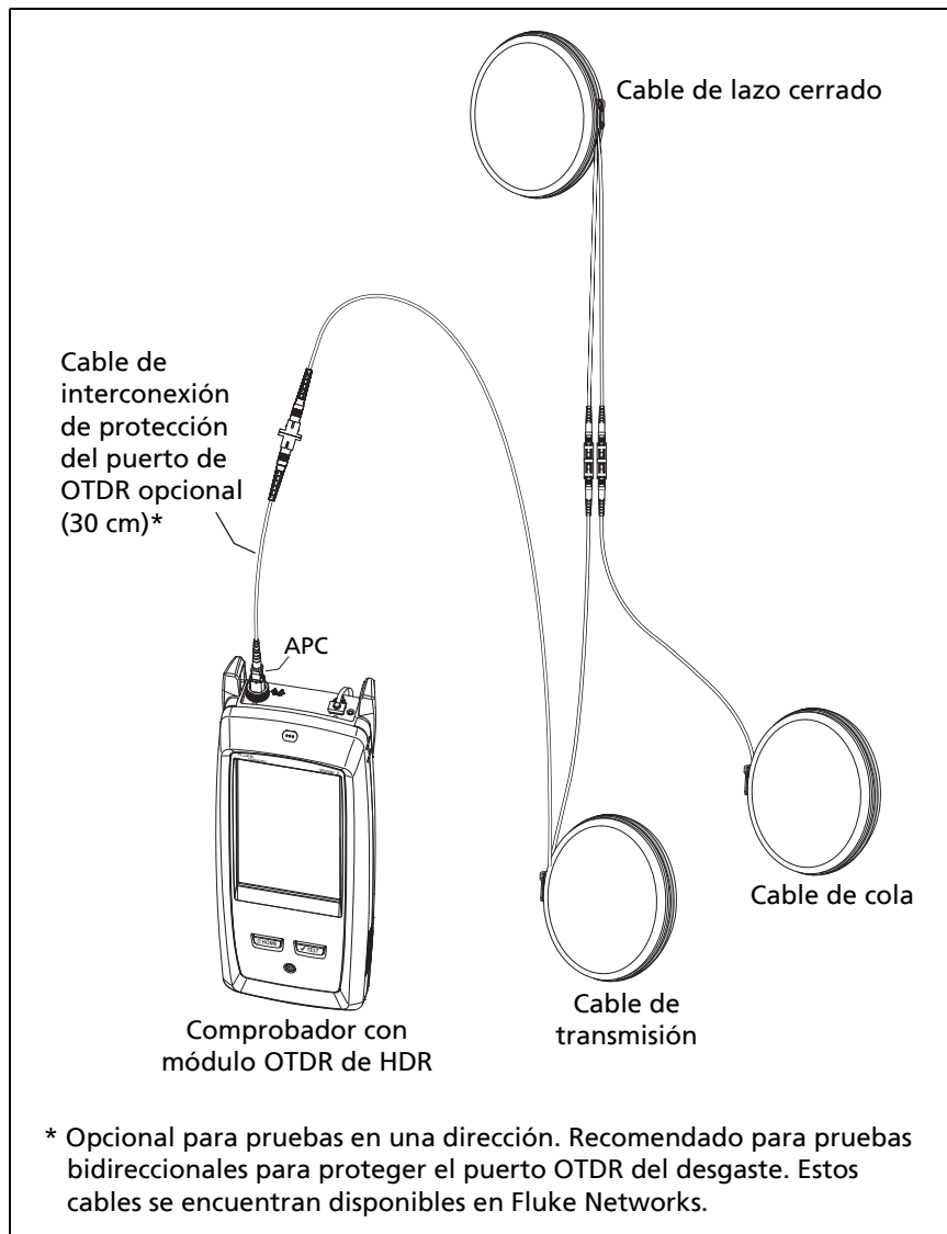
Figura 110. Conexiones de compensación de transmisión de SmartLoop
