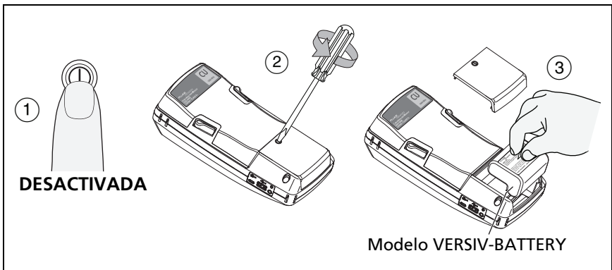
Figura 132. Cómo quitar la batería
