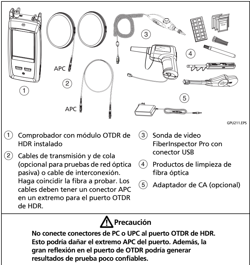
Figura 99. Equipo para pruebas de OTDR de HDR
