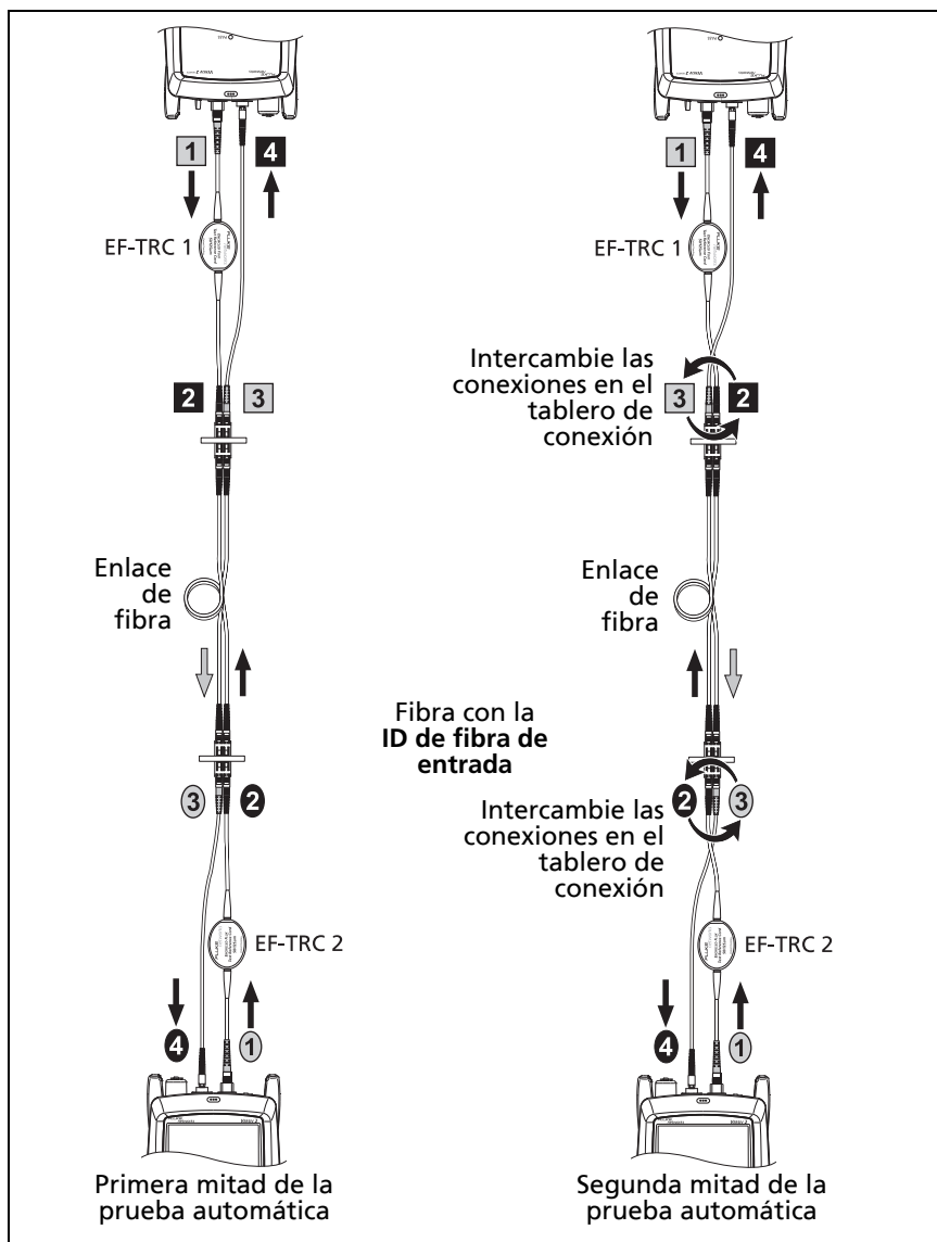
Figura 70. Conexiones para prueba bidireccional en modo remoto inteligente (referencia de 1 puente, fibra multimodal)
