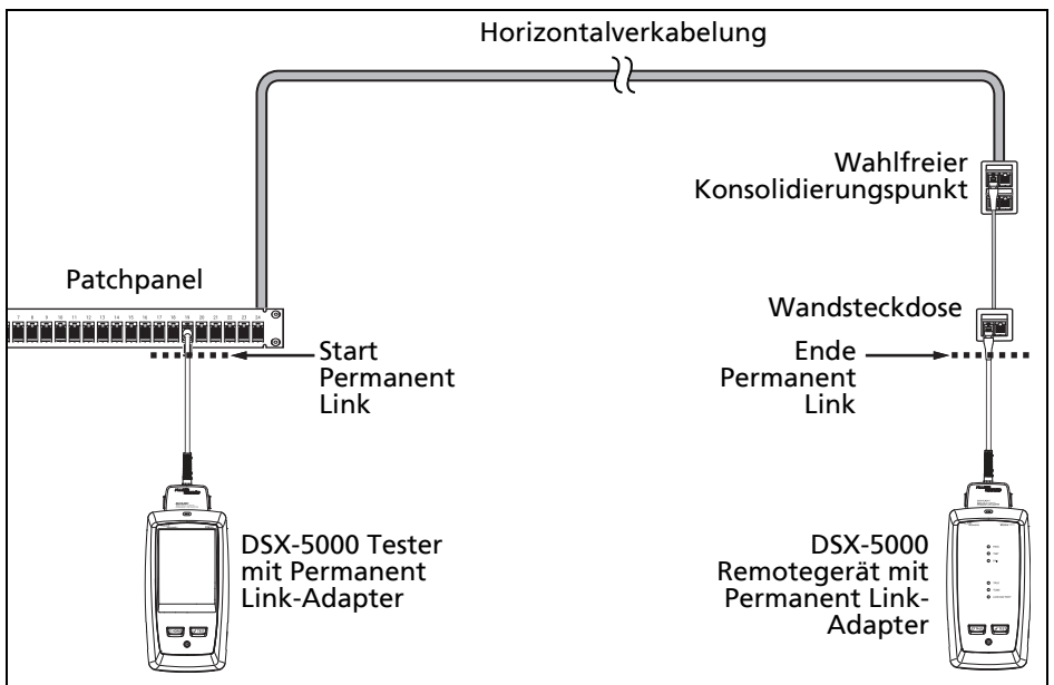
Abbildung 3. Permanent Link-Verbindungen
