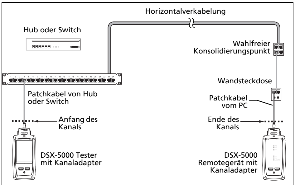
Abbildung 4. Kanalverbindungen (Abb. zeigt DSX-CHA-5-GG45 Kanaladapter)
