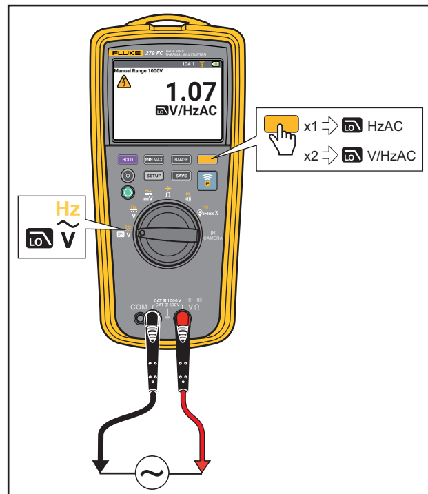
Figura 6. Relación de voltios/hercios
