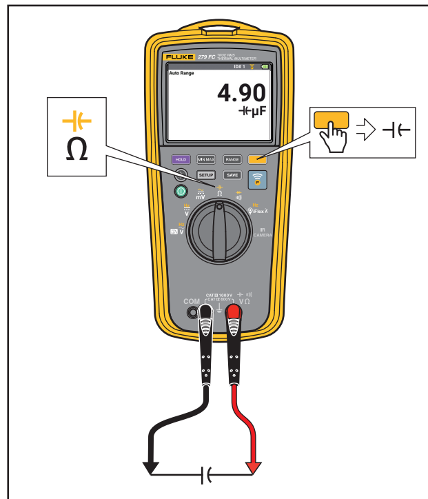
Figura 8. Mediciones de capacidad
