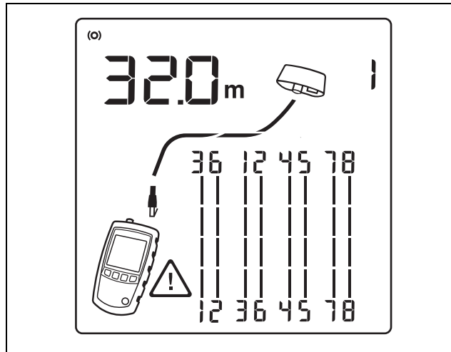
Figura 11. Pares cruzados
