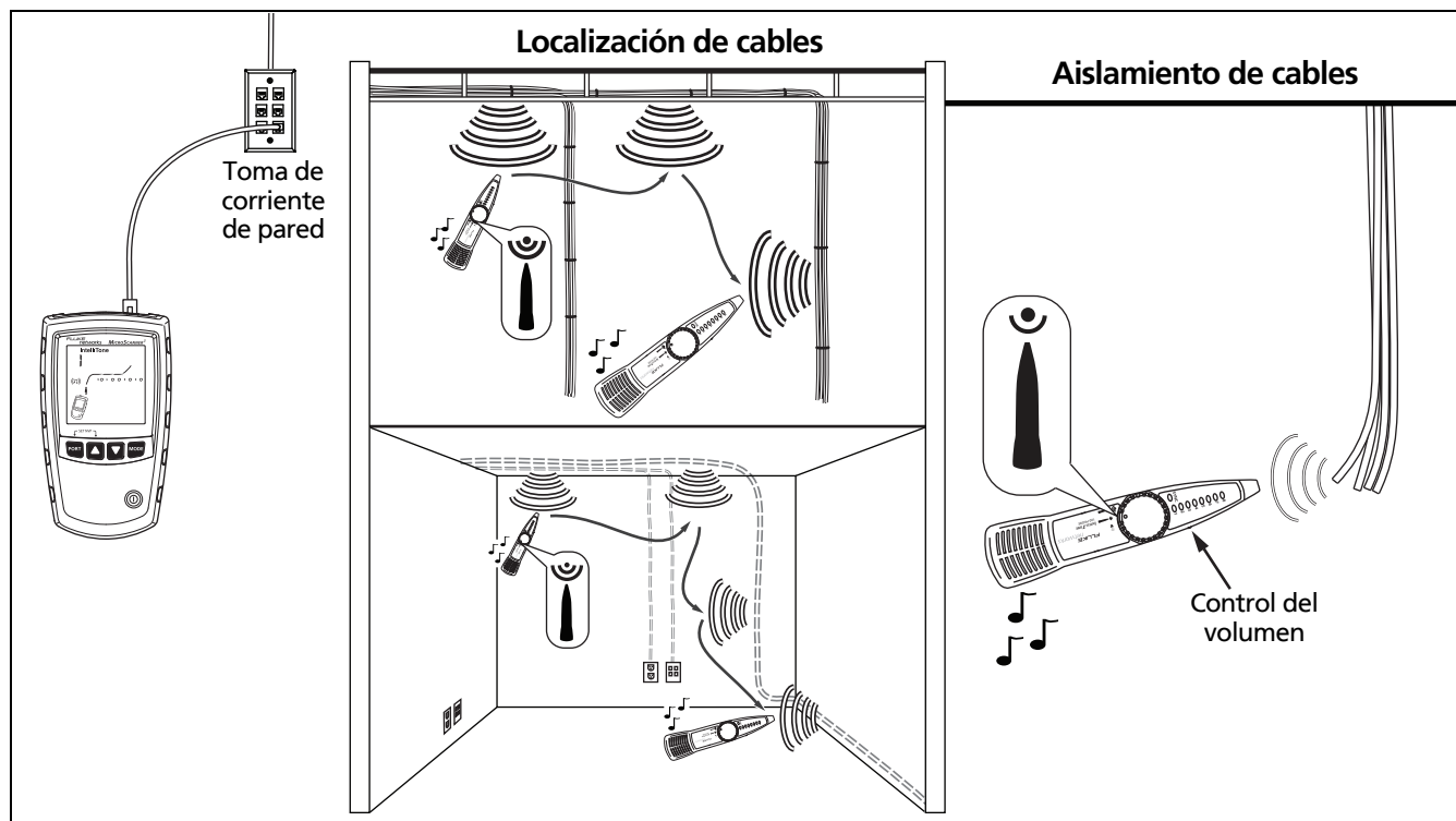
Figura 34. Utilización del emisor de tonos en el modo IntelliTone
