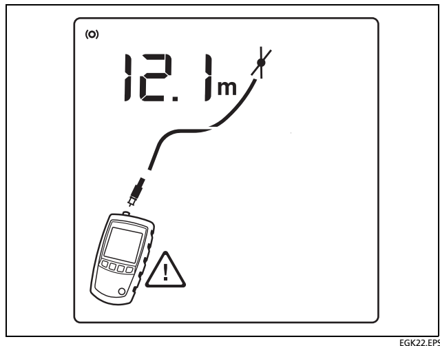
Figura 25. Cortocircuito en cableado coaxial (MicroScanner²)
