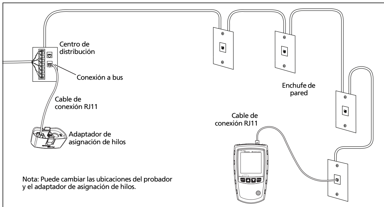
Figura 21. Conexión a una red telefónica cableada en una topología de bus
