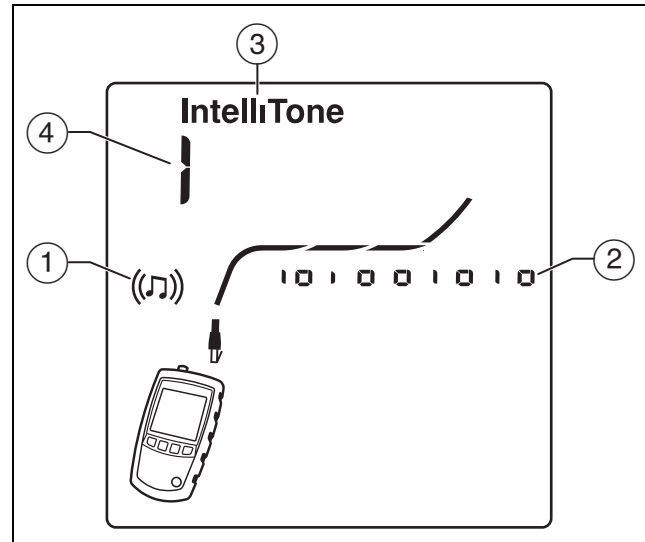
Abbildung 33. IntelliTone Toner-Modusanzeige
