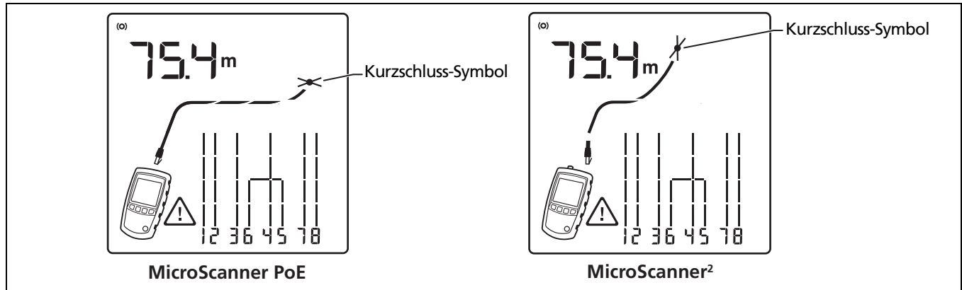
Abbildung 9. Kurzschluss in Twisted-Pair-Verkabelung
