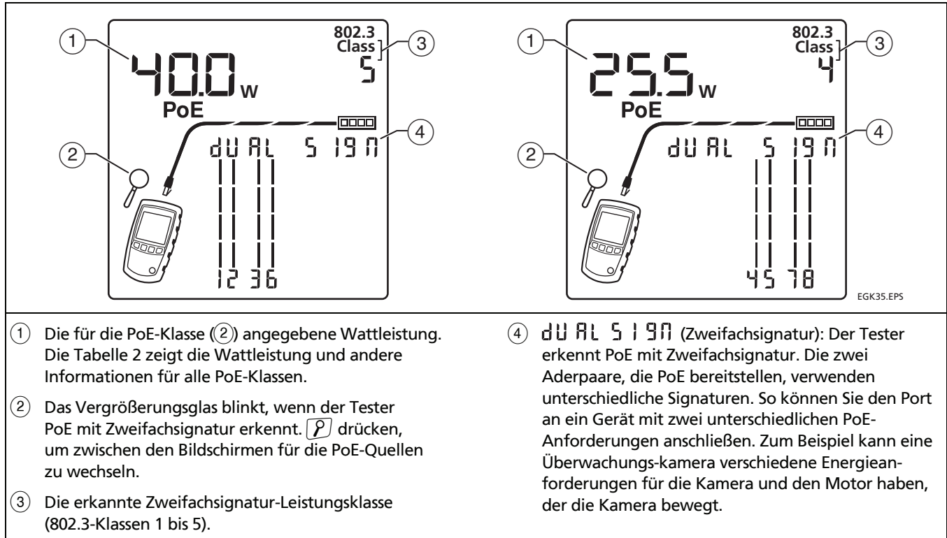
Abbildung 30. Detailanzeige der PoE-Klassen 5 und 4 von einer Quelle mit Zweifachsignatur (MicroScanner PoE)
