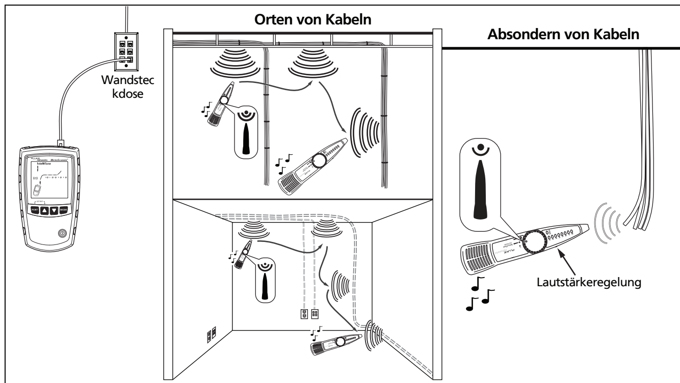
Abbildung 34. Verwenden des Toners im IntelliTone-Modus
