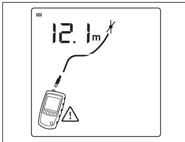
Abbildung 25. Kurzschluss in Koaxialkabel (MicroScanner 2 )
