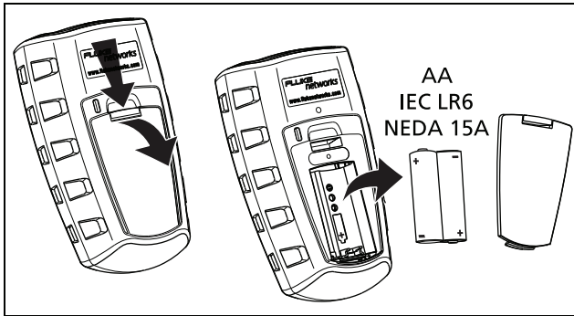
Abbildung 37. Ersetzen der Batterien des Testers
