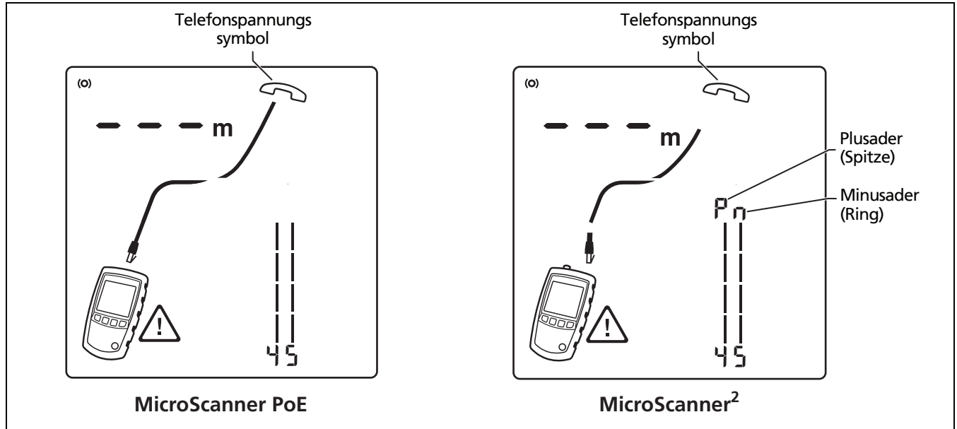
Abbildung 13. Telefonspannungen erkannt
