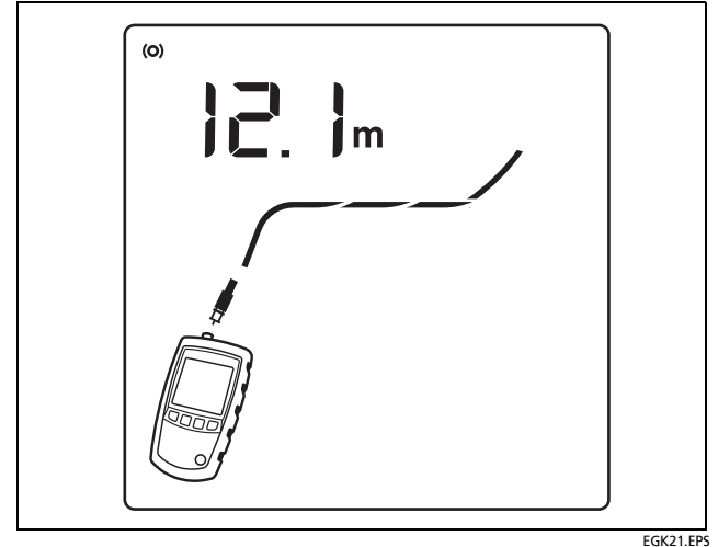
Abbildung 24. Offene Stelle auf Koaxialkabel (MicroScanner 2 )
