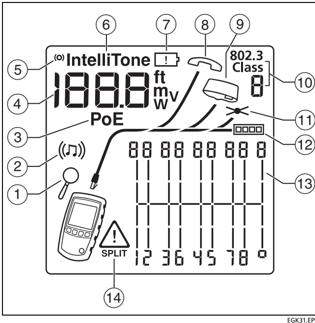
Abbildung 3. MicroScanner PoE-Anzeigefunktionen
