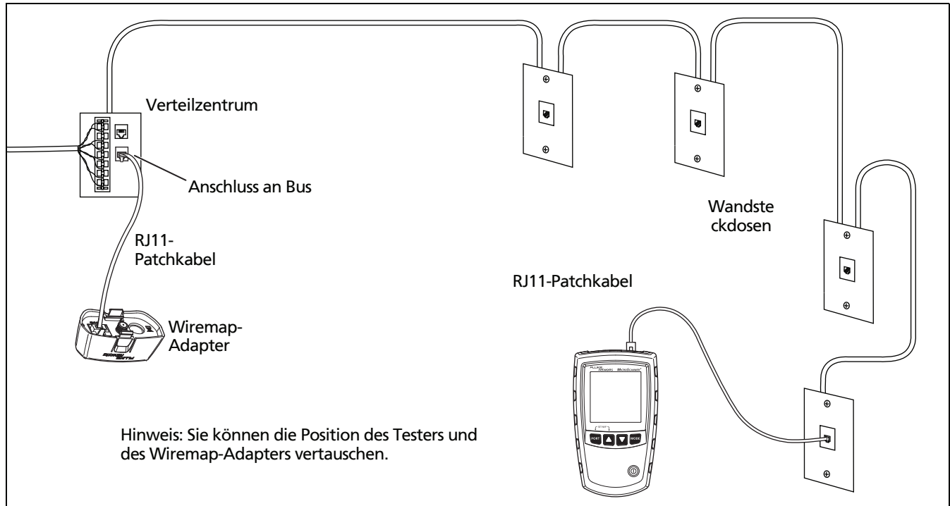
Abbildung 21. Anschließen an ein Telefonnetz in einer Bustopologie
