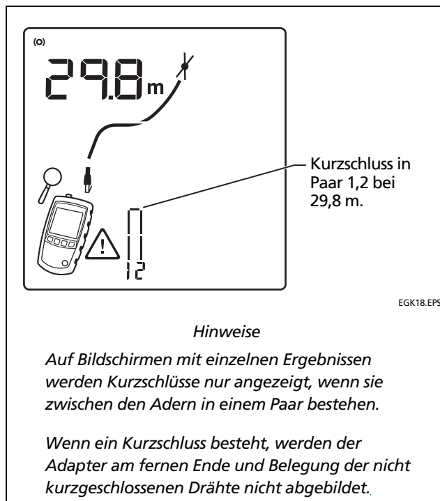
Abbildung 17. Details für einen Kurzschluss (MicroScanner 2 -Bildschirm dargestellt)
