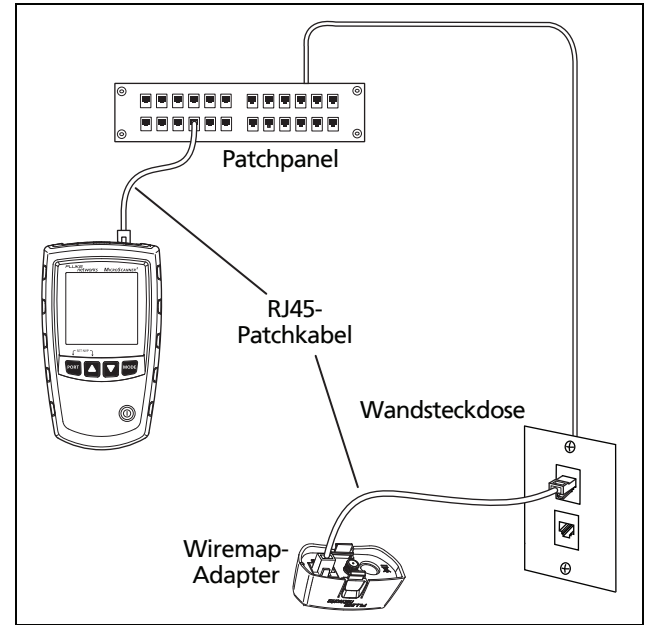
Abbildung 7. Anschließen an eine Twisted-Pair-Netzwerkverkabelung
