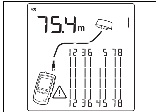
Abbildung 8. Offener Schaltkreis auf Twisted-Pair-Verkabelung
