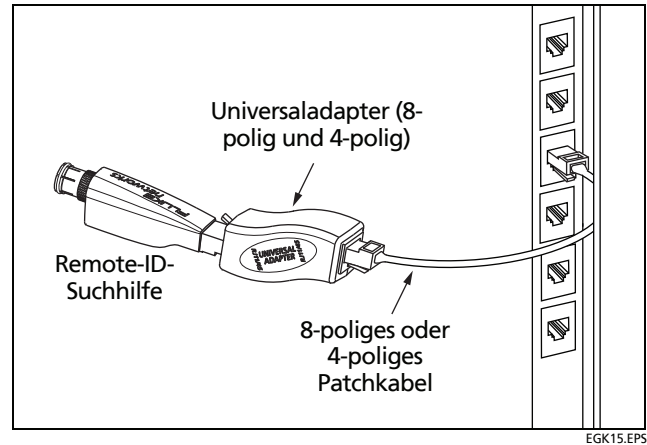
Abbildung 6. Anschließen einer Remote-ID-Suchhilfe an einen modularen Stecker in einem geschlossenen Bereich oder an einen RJ11-Stecker
