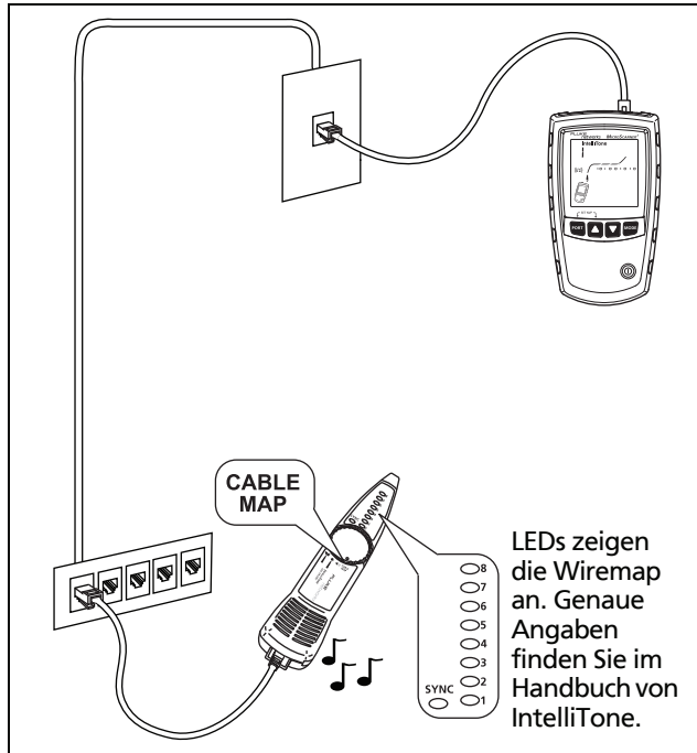
Abbildung 36. Verwendung des Toners mit der IP200 IntelliTone-Kabelbelegungsfunktion
