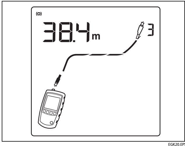
Abbildung 23. Koaxialergebnisse (MicroScanner 2 )
