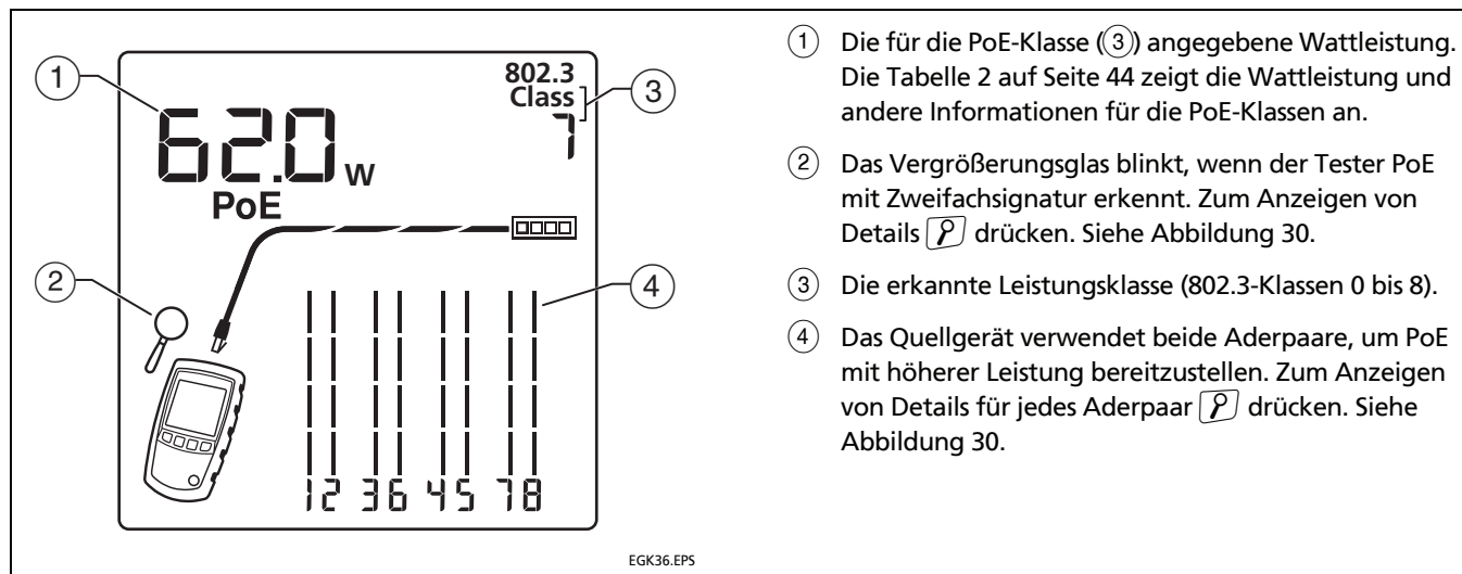
Abbildung 29. PoE aus einer Zweifachsignatur-PoE-Quelle (MicroScanner PoE)
