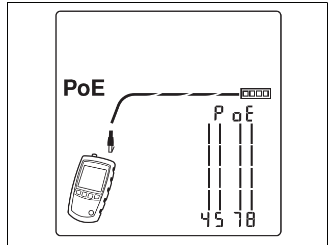
Abbildung 27. MicroScanner 2 PoE-Anzeige
