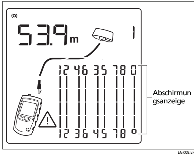
Abbildung 10. Gekreuzte Drähte
