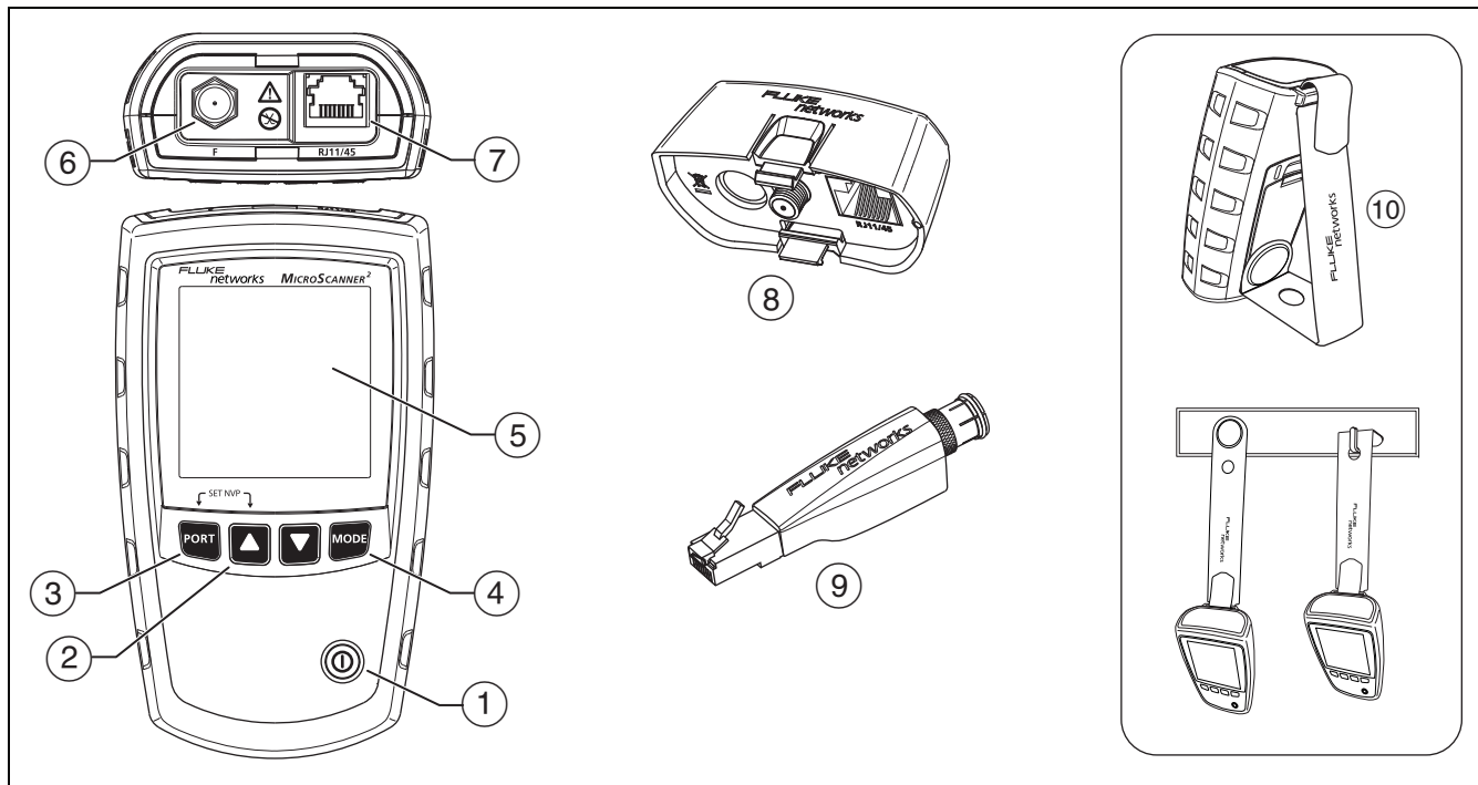
Abbildung 4. MicroScanner 2 Merkmale
