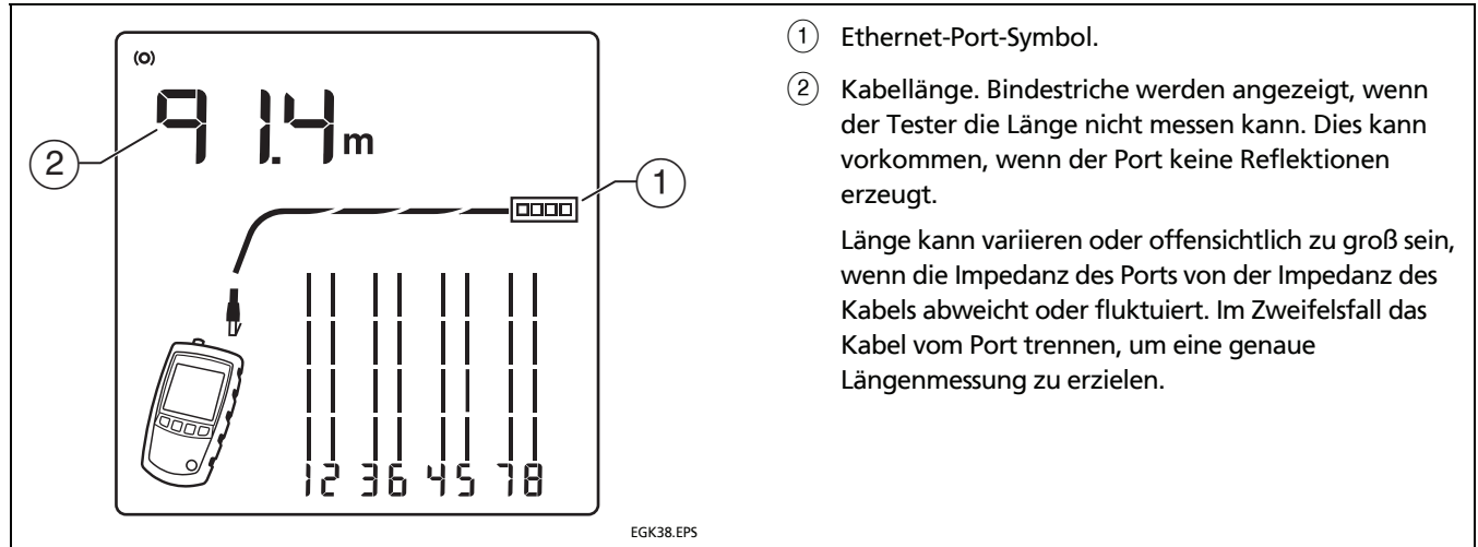
Abbildung 16. Inaktiver Ethernet-Port erkannt
