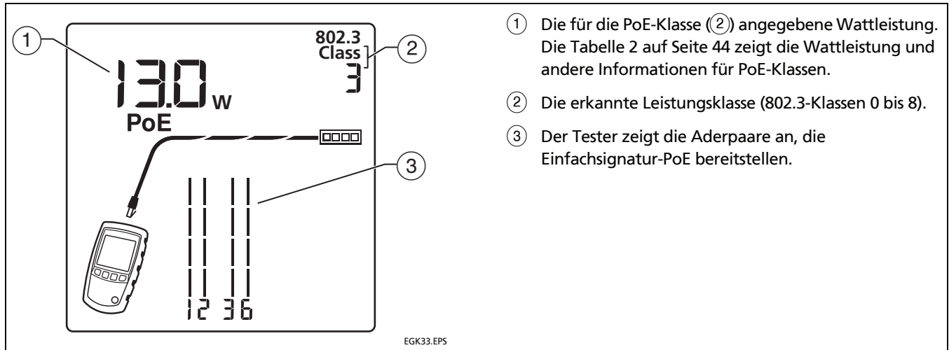
Abbildung 28. PoE aus einer Quelle, die nur Einfachsignatur-PoE (MicroScanner PoE) bereitstellt
