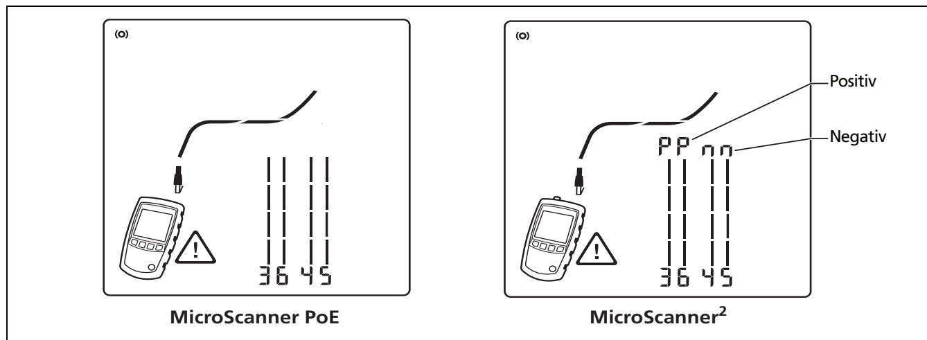
Abbildung 1. Anzeigebeispiele für Hochspannung
