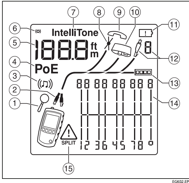
Abbildung 5. MicroScanner 2 -Anzeigefunktionen
