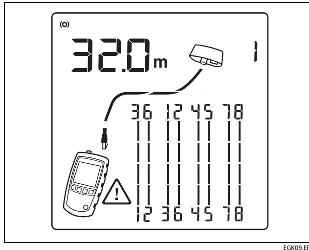
Abbildung 11. Gekreuzte Paare
