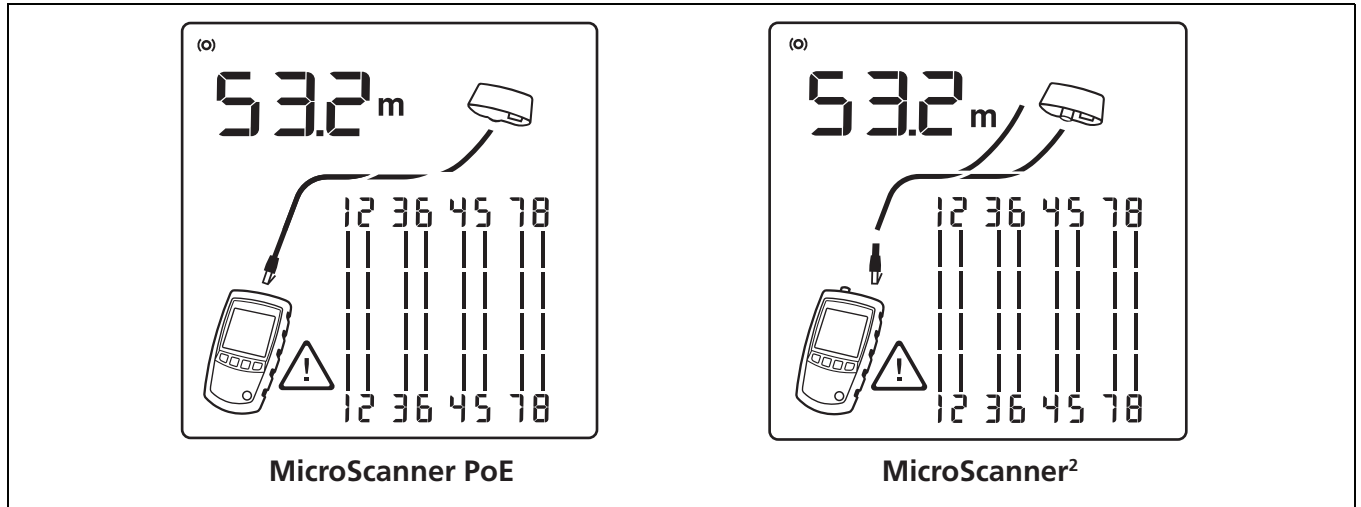
Abbildung 14. Stichleitung erkannt
