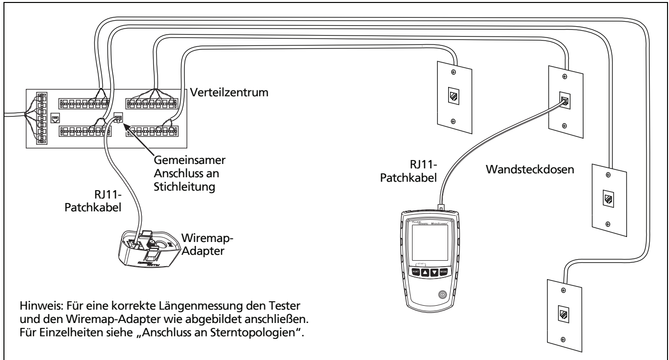
Abbildung 20. Anschließen an ein Telefonnetz in einer Sterntopologie
