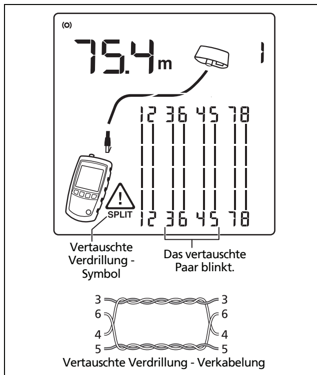
Abbildung 12. Vertauschte Verdrillung
