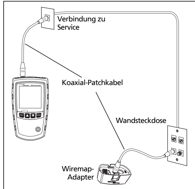
Abbildung 22. Anschließen an Koaxialkabel (MicroScanner 2 )
