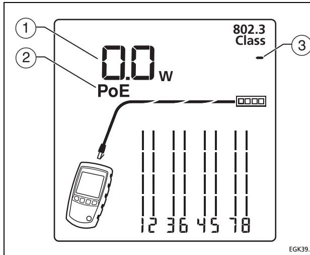
Abbildung 31. PoE-Port, für den „0.0 W“ angezeigt wird
