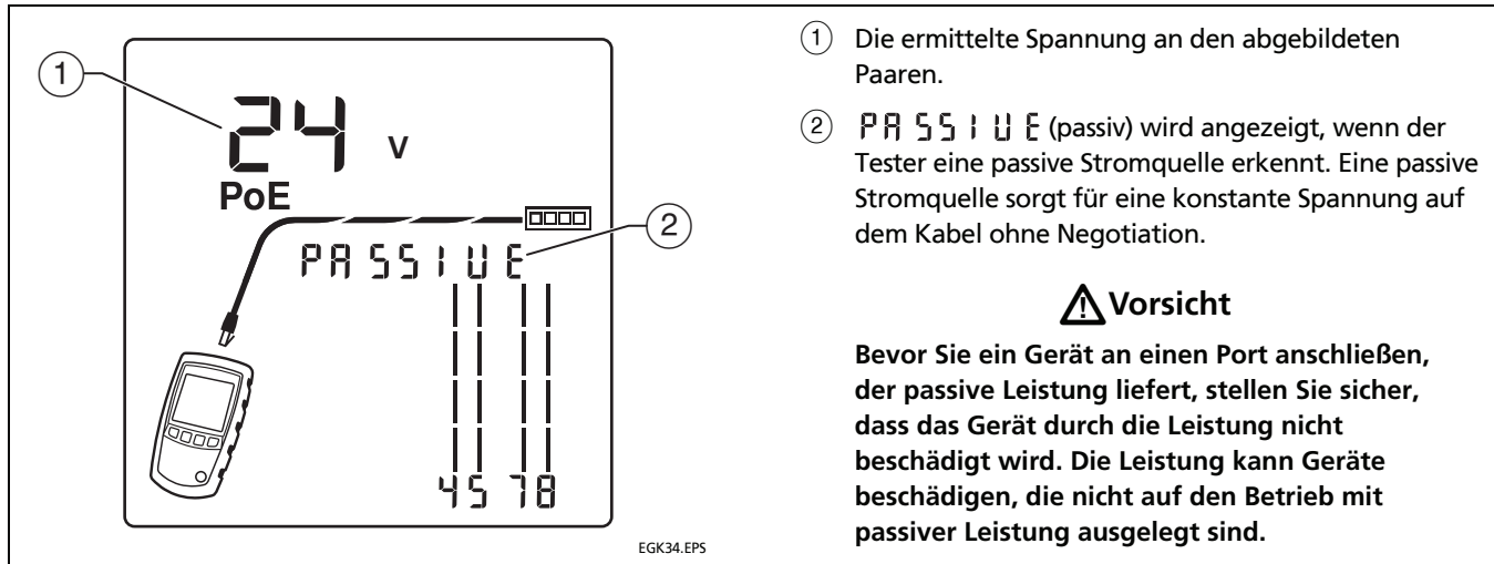
Abbildung 32. Passive Leistung (MicroScanner PoE)
