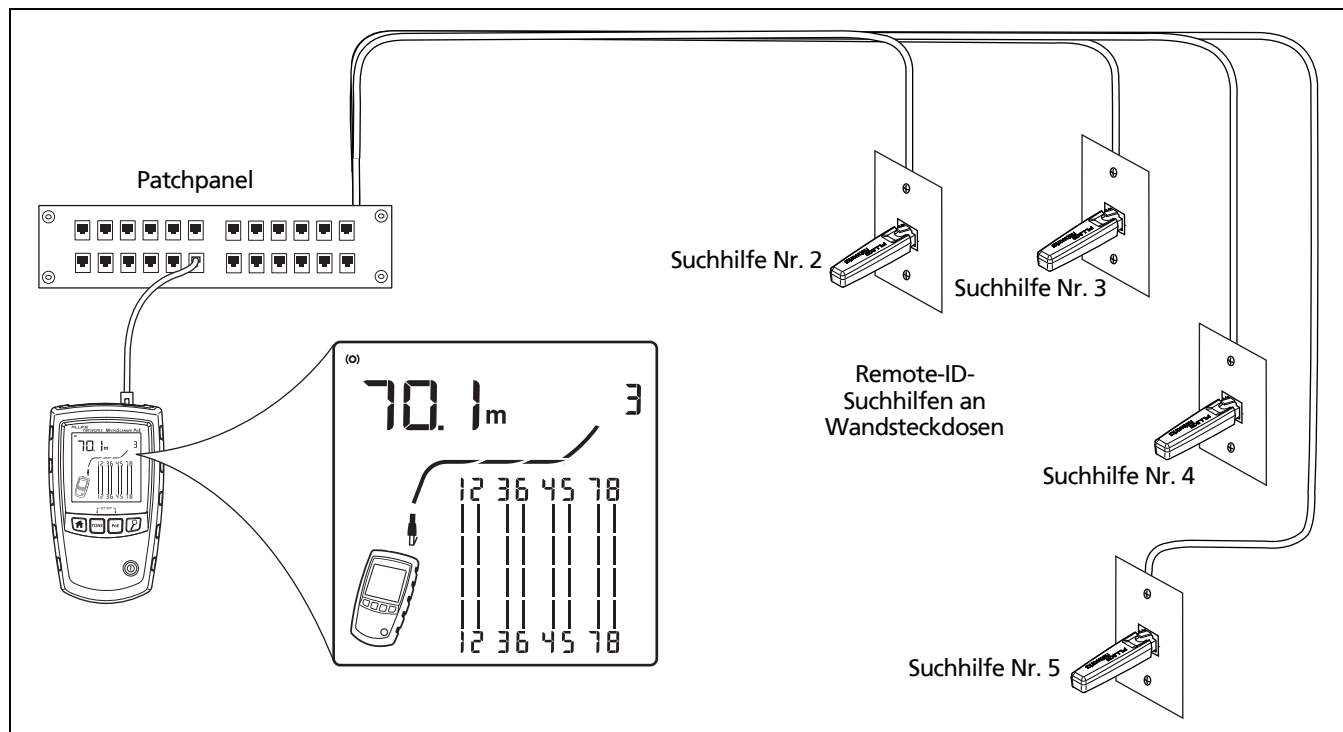
Abbildung 19. Verwenden mehrerer Remote-ID-Suchhilfen (MicroScanner PoE abgebildet)
