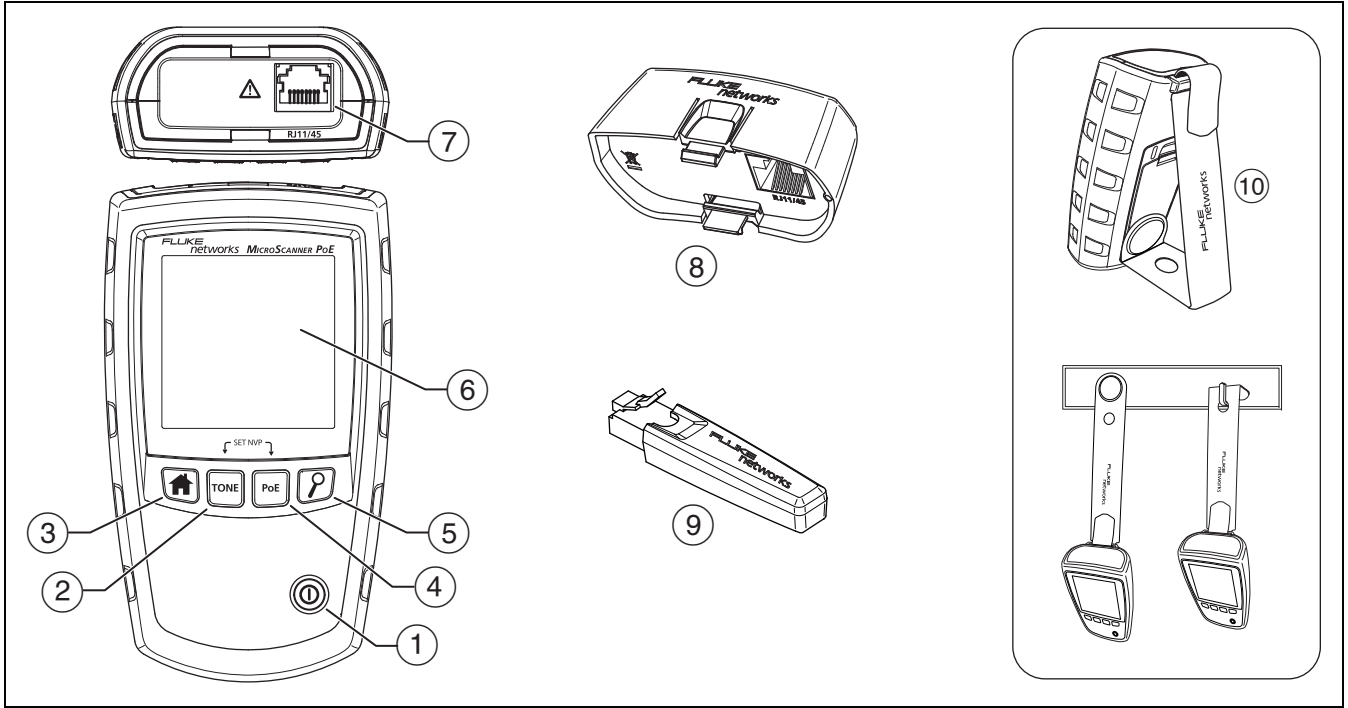
Abbildung 2. MicroScanner PoE-Funktionen
