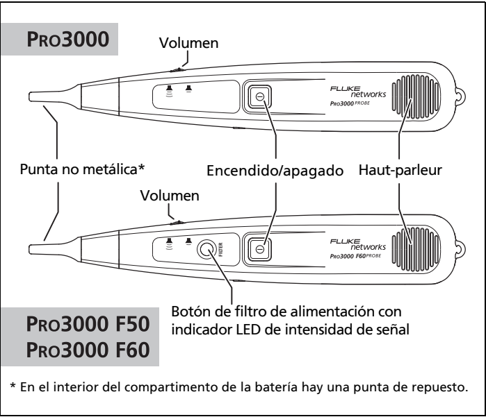
Figura 1. Sondas PRO3000, PRO3000 F50, y PRO3000 F60
