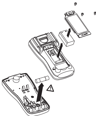
Rysunek 2. Demontaż
