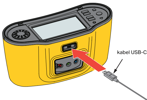
Obrázek 27. Připojení kabelu USB-C
