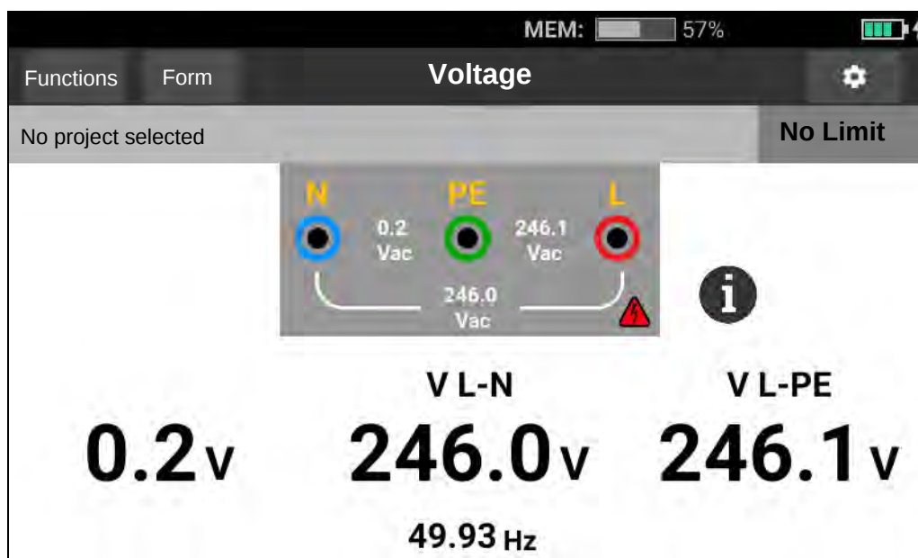
Obrázek 8. Obrázovka měření napětí a frekvence
