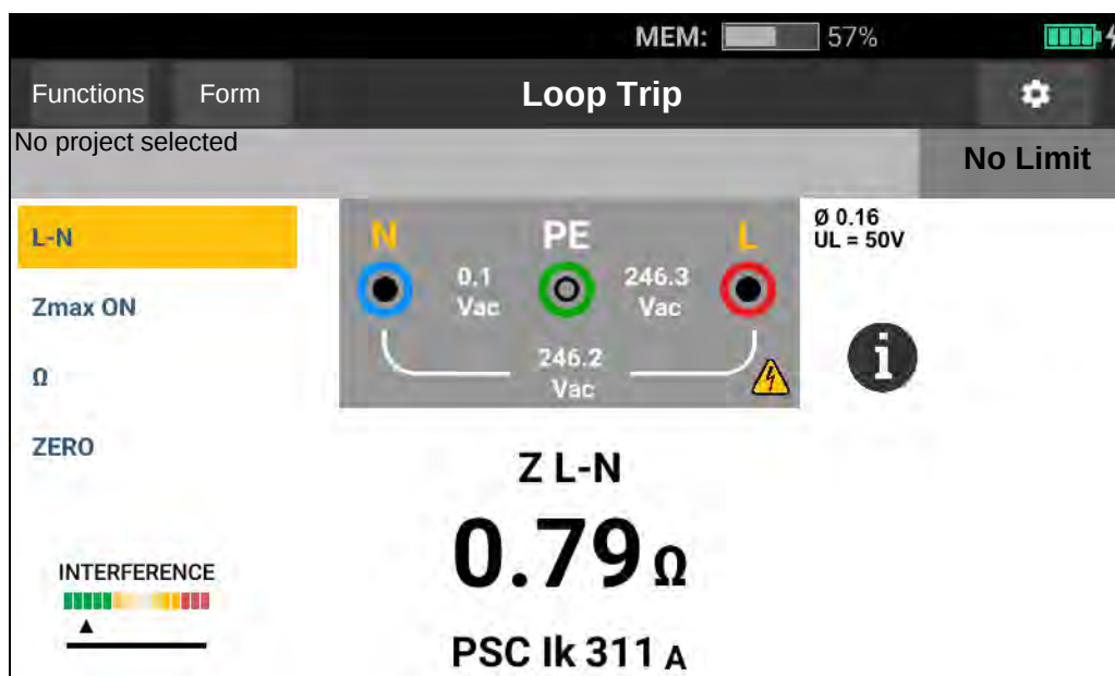
Obrázek 13. Obrázovka měření impedance sítě
