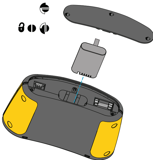
Obrázek 28. Výměna baterie
