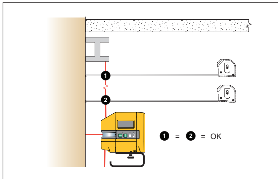
Figura 6. Verifica del livellamento verticale di un elemento esistente
