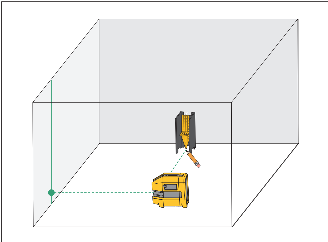
Figura 7. Nuovo angolo retto
