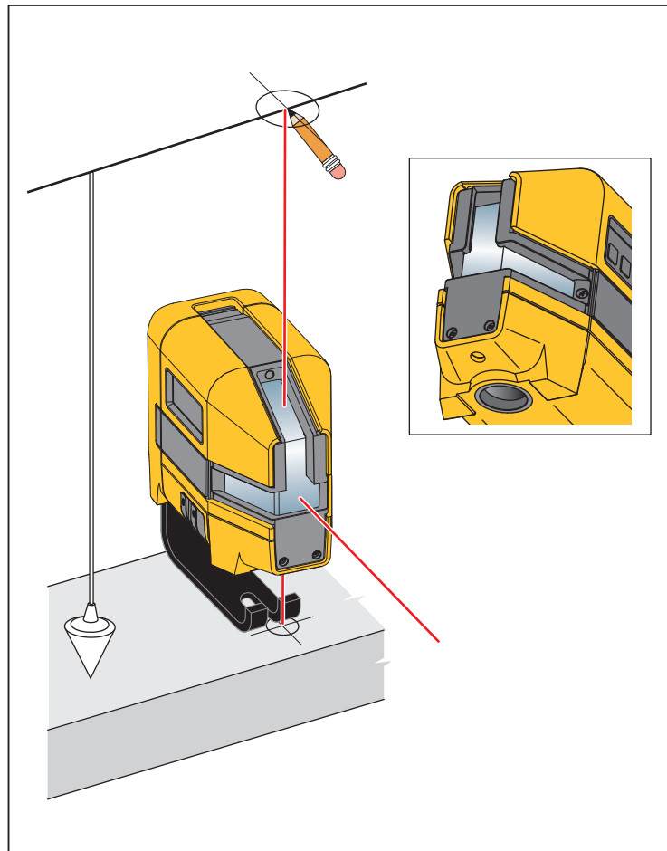
Figura 5. Nuovo contrassegno verticale
