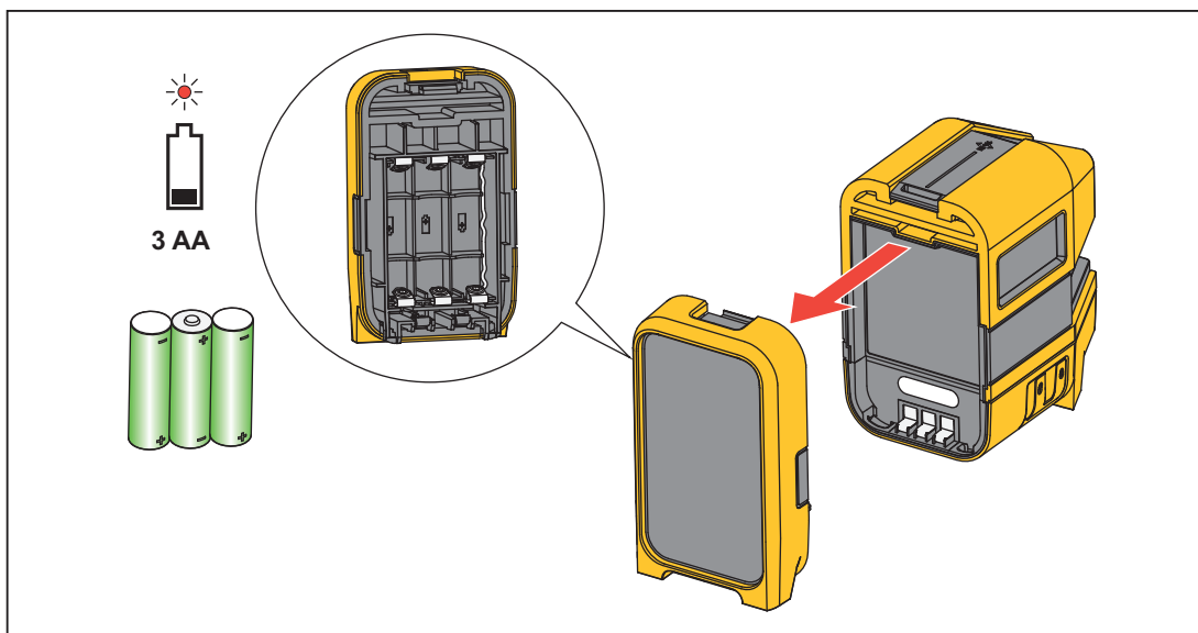
Figura 11. Sostituzione delle pile
