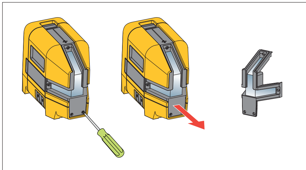
Figura 12. Sostituzione dell'inserto alloggiamento in vetro
