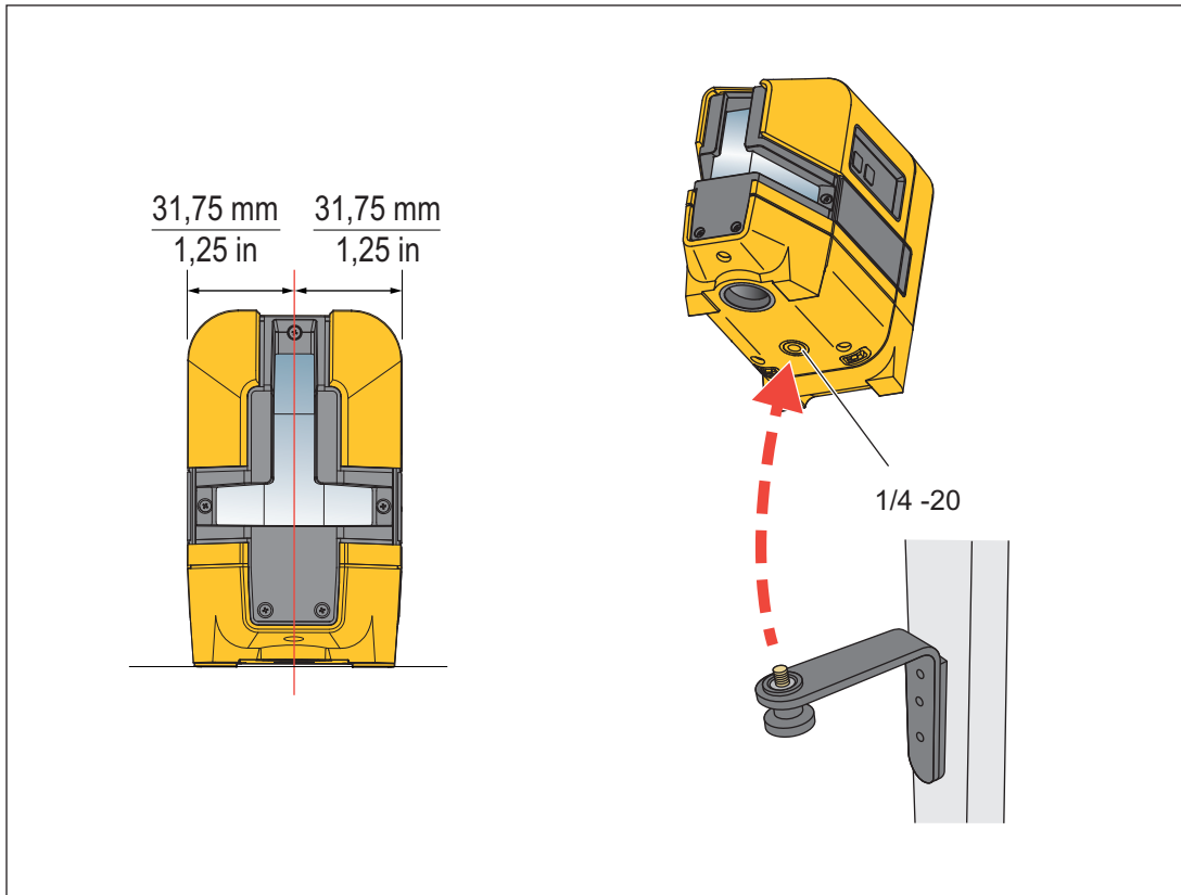
Figura 1. Punto centrale e supporto accessorio
