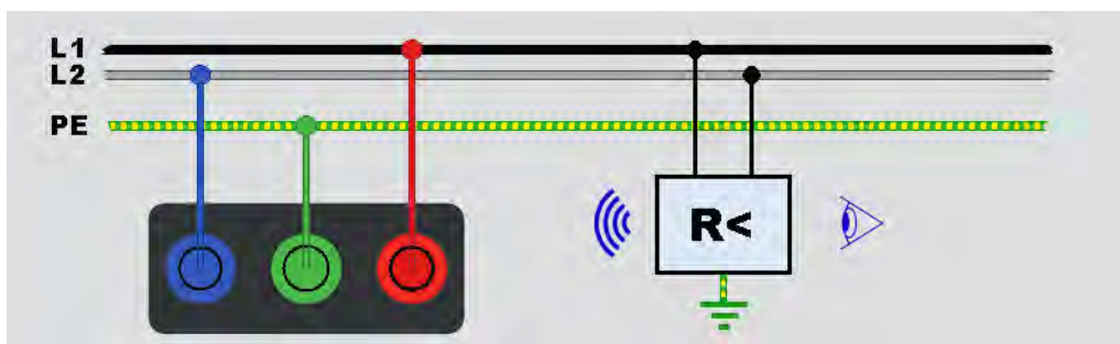
Figura 23. Prueba de IMD n.º 1
