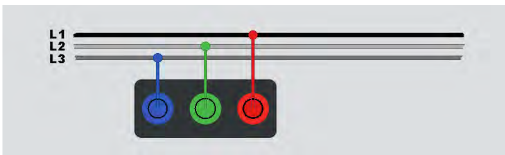
Figura 19. Conexión para prueba de rotación de fases
