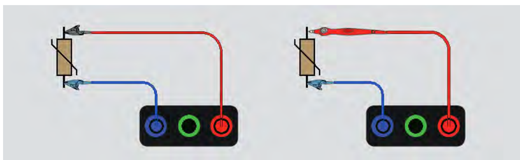
Figura 22. Conexión para prueba de SPD
