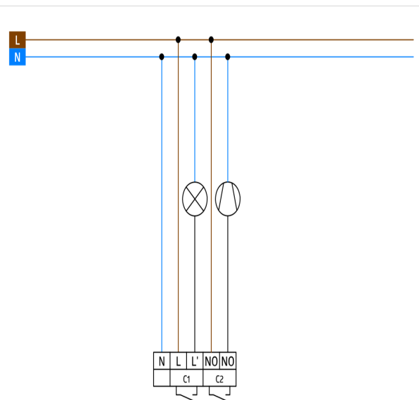
Wiring diagramms
