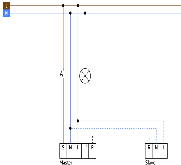
Wiring diagrams
