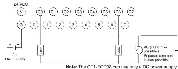
GT1-ROP08/GT1-FOP08
