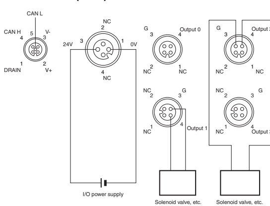
DRT2-OD04CL-1 (PNP)
