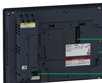
Vue arrière du HMIDT65X
