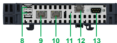
Vue de dessous du HMIG3X
