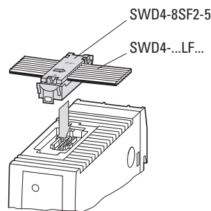
Abbildung 96: SWD-Koordinator an PXR-RCAM-SWD anschließen
