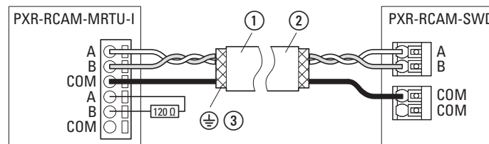
Abbildung 97: Verdrahtung
