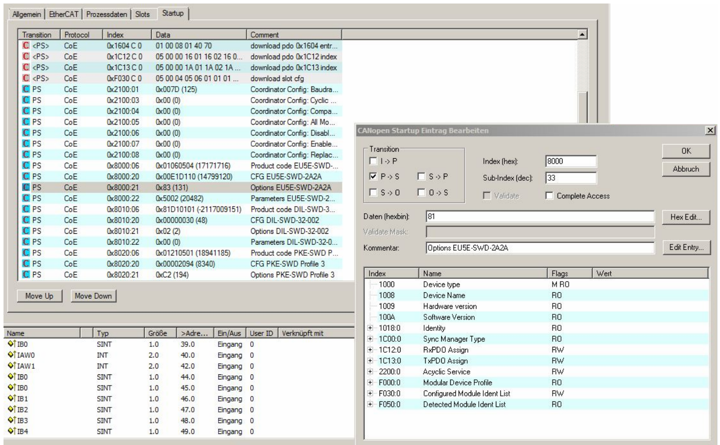
Abbildung 98: Ändern des Optionsbytes beim Modul EU5E-SWD-2A2A
