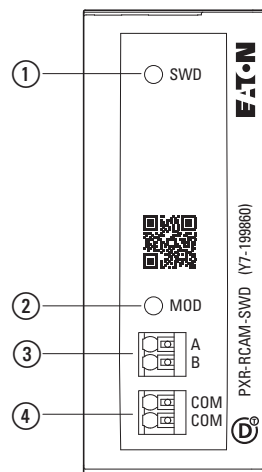
Abbildung 90: Frontseite PXR-RCAM-SWD
