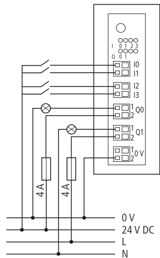
Abbildung 17: Anschluss der Ein-/Ausgänge des Moduls EU5E-SWD-4D2R
