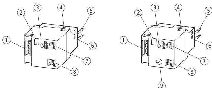
Abbildung 27: Anschlüsse des SmartWire-DT Moduls DIL-SWD-32-001 bzw. DIL-SWD-32-002 für DILM
