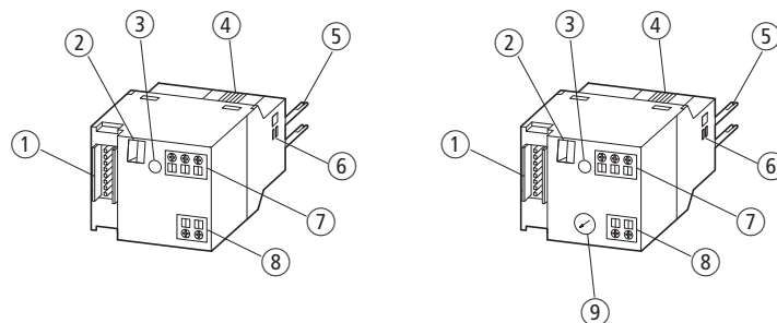
Abbildung 26: Aufbau der SmartWire-DT Module DIL-SWD-32-001 und DIL-SWD-32-002 für DILM
