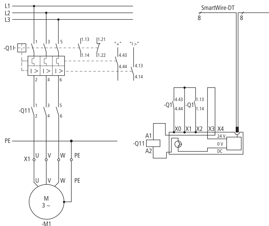
Abbildung 28: Stromlaufplan des Direktstarters
