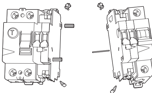
Abbildung 78: Verbindungsbolzen entfernen
