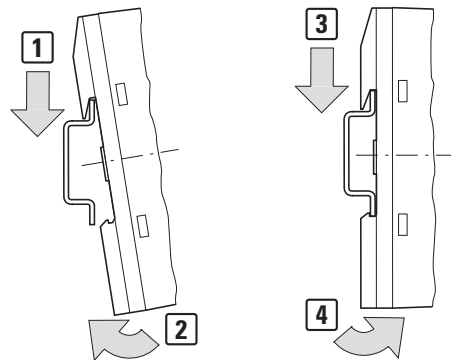
Abbildung 91: PXR-RCAM-SWD montieren
