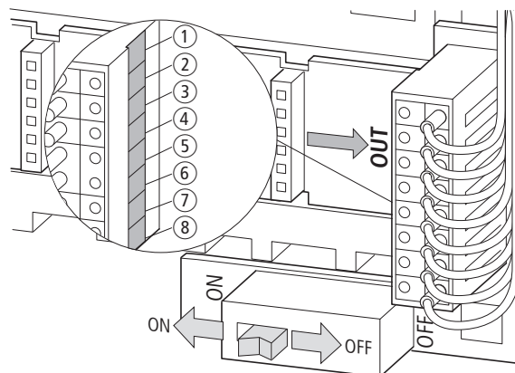
Abbildung 67: Abschlusswiderstand
