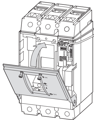
Abbildung 95: NZM schließen
