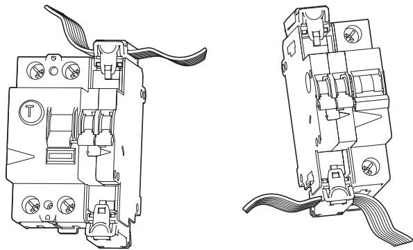
Abbildung 79: Anschluss der SmartWire-DT Leitung
