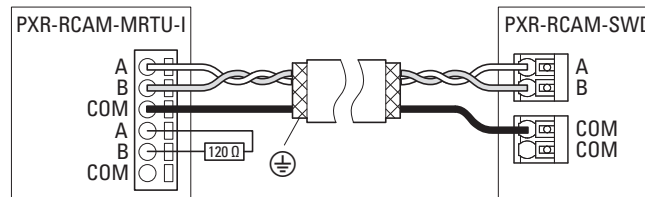
Abbildung 93: PXR-RCAM-SWD an den Leistungsschalter anschließen
