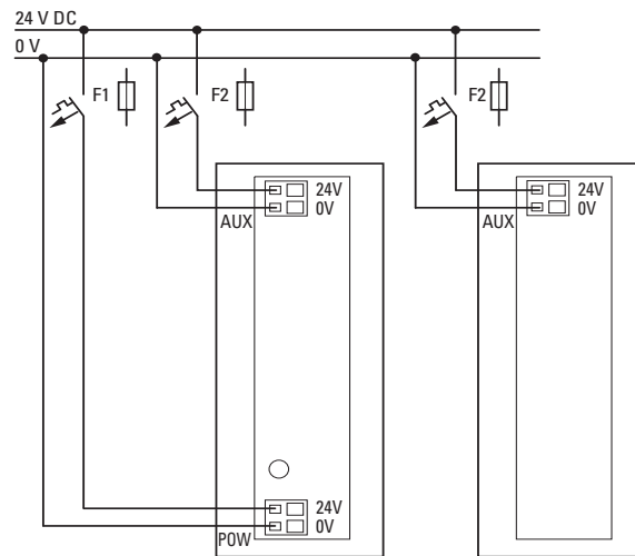
Abbildung 4: Anschlussquerschnitte
