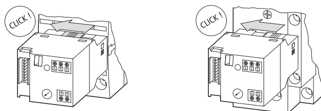
Abbildung 37: Verriegeln des DIL-SWD-32-001 bzw. des DIL-SWD-32-002
