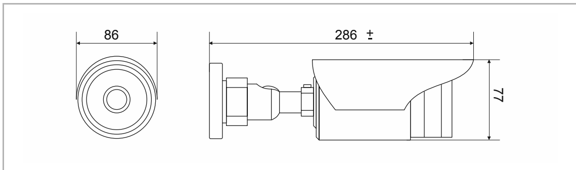
Abb. 1: Abmessungen
