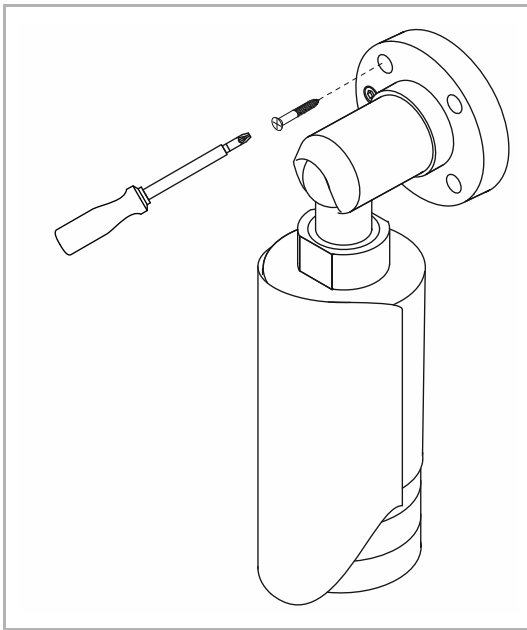
Abb. 4: Kamera geschwenkt
