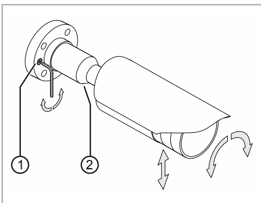
Abb. 3: Kamerawinkel einstellen
