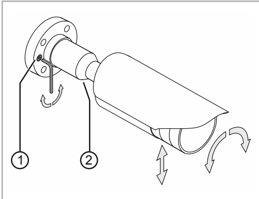
Abb. 9: Kamerawinkel einstellen
