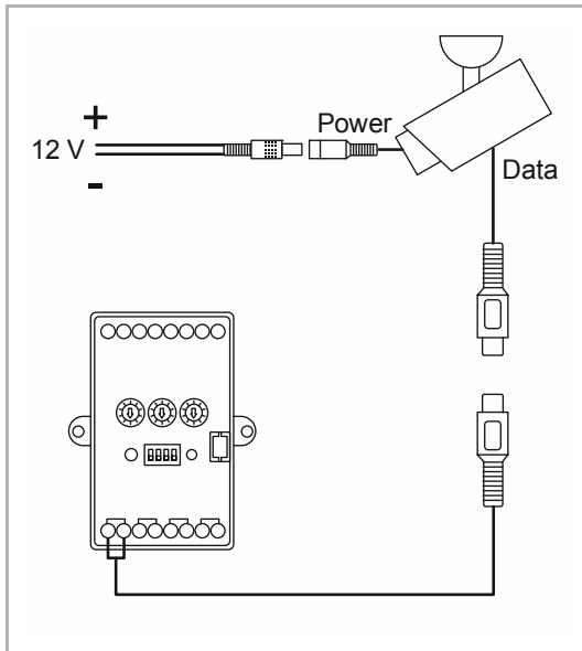
Abb. 6: Elektrischer- und Multimedia-Anschluss (permanente Spannungsversorgung)
