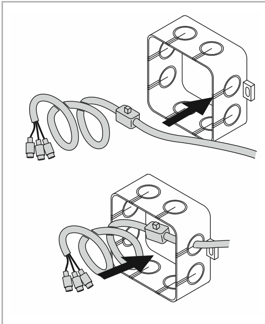
Abb. 5: Beispiel: Anschlussdose
