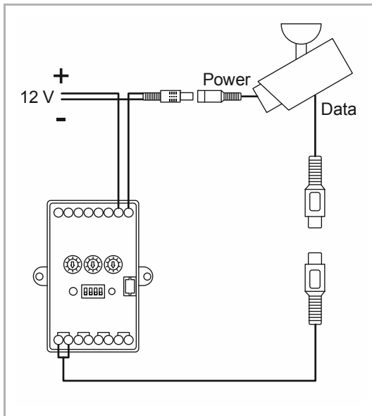
Abb. 7: Elektrischer- und Multimedia-Anschluss (Nicht-permanente Spannungsversorgung)
