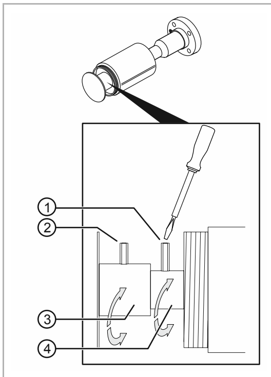
Abb. 12: Fokus und Zoom einstellen
