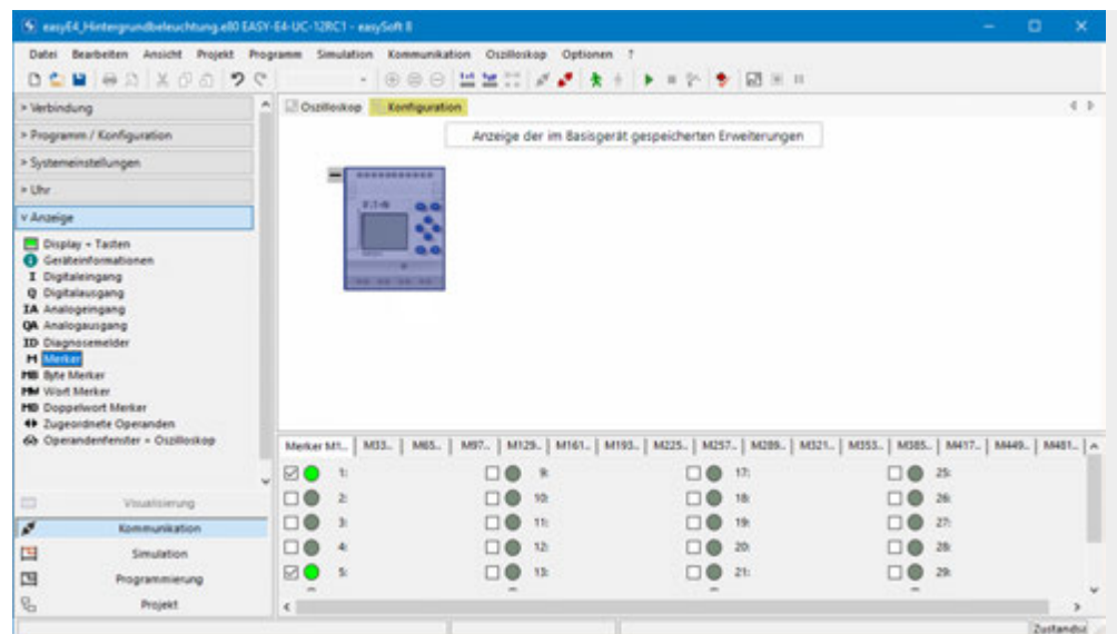
Abb. 305: Ansicht Kommunikation ONLINE mit Anzeige Merker; das Gerätedisplay blinkt grün
