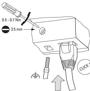
Abb. 37: Ethernet-Leitung anschließen
