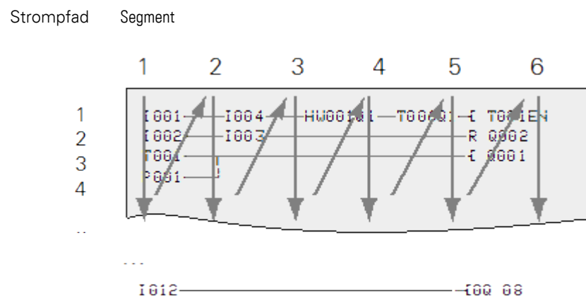
Abb. 303: Wie easyEDP Schaltplan und Funktionsbausteine ausgewertet
