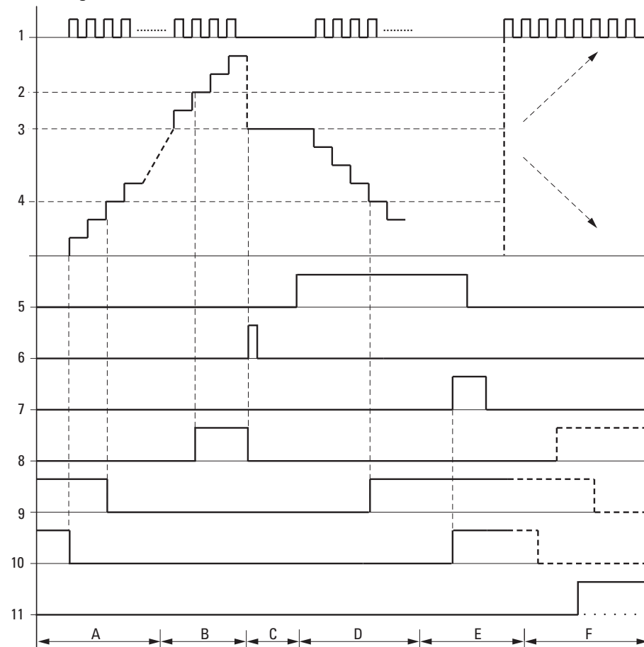
Abb. 174: Wirkdiagramm Hochgeschwindigkeitszähler
