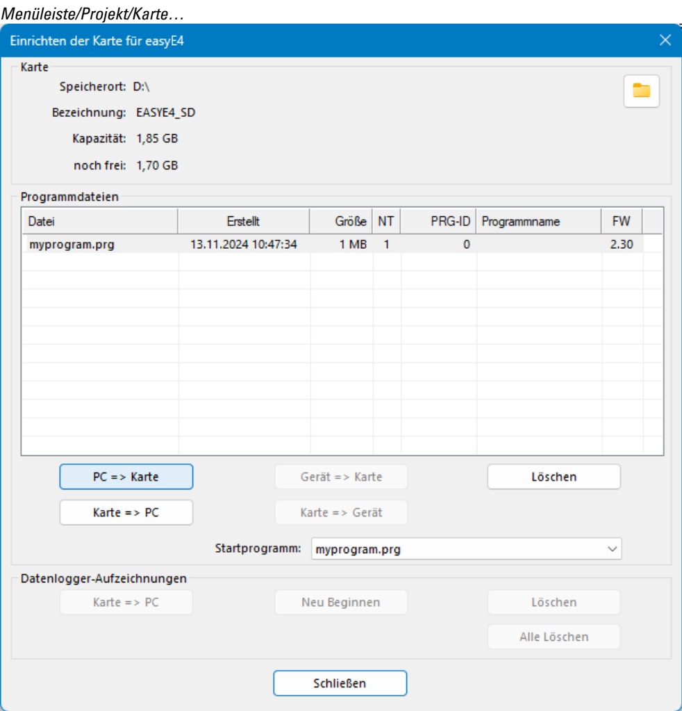
Abb. 72: Offline Bediendialog Speicherkarte
