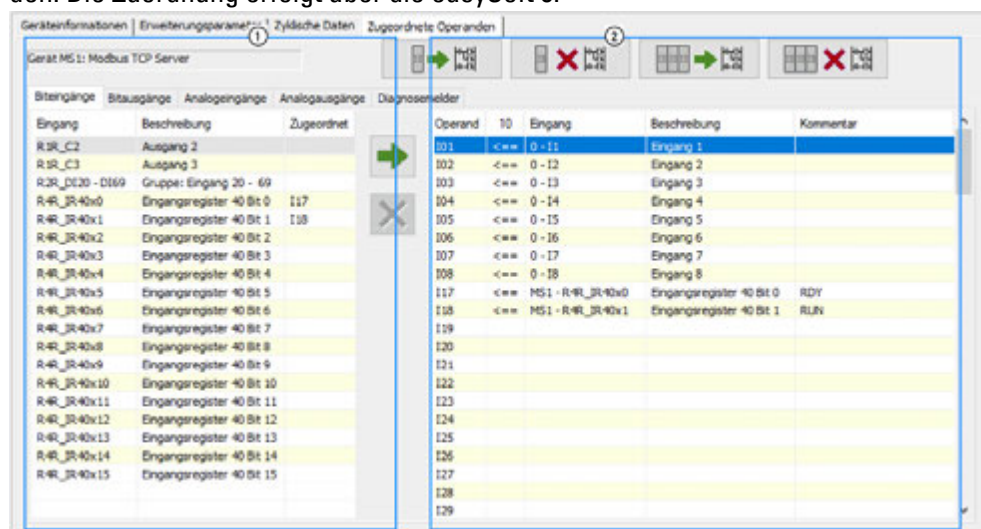
Abb. 390: Register Zugeordnete Operanden nach Definition von FC1, FC2 und FC4; Biteingänge R4R_ IR40x0 und R4R_ IR40x1 wurden den Operanden des Basisgerätes I17 und I18 bereits zugeordnet.
