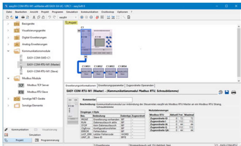
Abb. 352: Arbeitsfläche mit Basisgerät und Kommunikationsmodul EASY-COM-RTU-M1 Master
