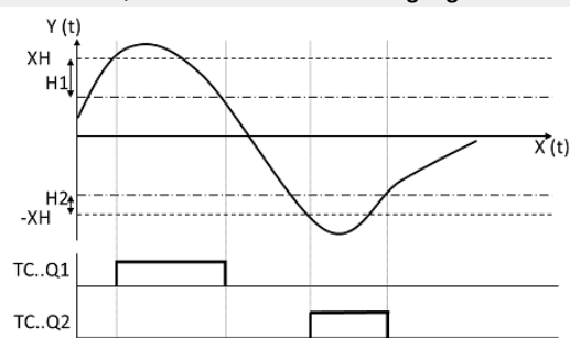
Abb. 205: Wirkdiagramm Dreipunktregler
