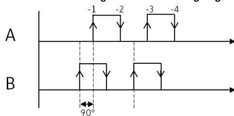
Abb. 176: Funktionsbaustein CI rückwärts zählend; QV=QV-4
