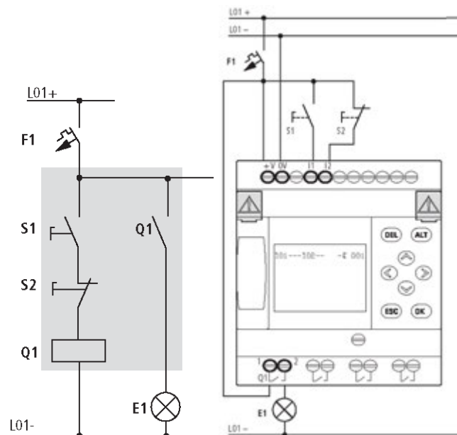
Abb. 83: Lampensteuerung
