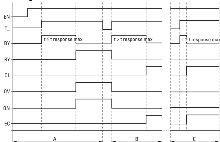
Abb. 242: Wirkdiagramm Frequenzzähler
