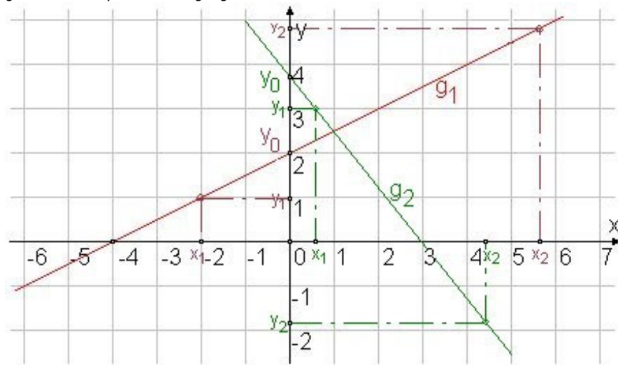
Abb. 187: Mathematischer Zusammenhang
