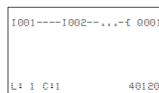
Abb. 84: Schaltplan mit Eingängen I01, I02 und Ausgang Q1
