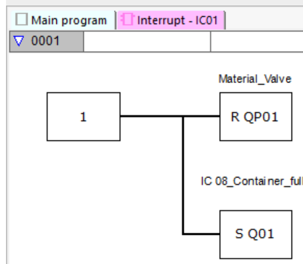
Abb. 261: easySoft 8 Interrupt-Programm zwei Zählereingänge
