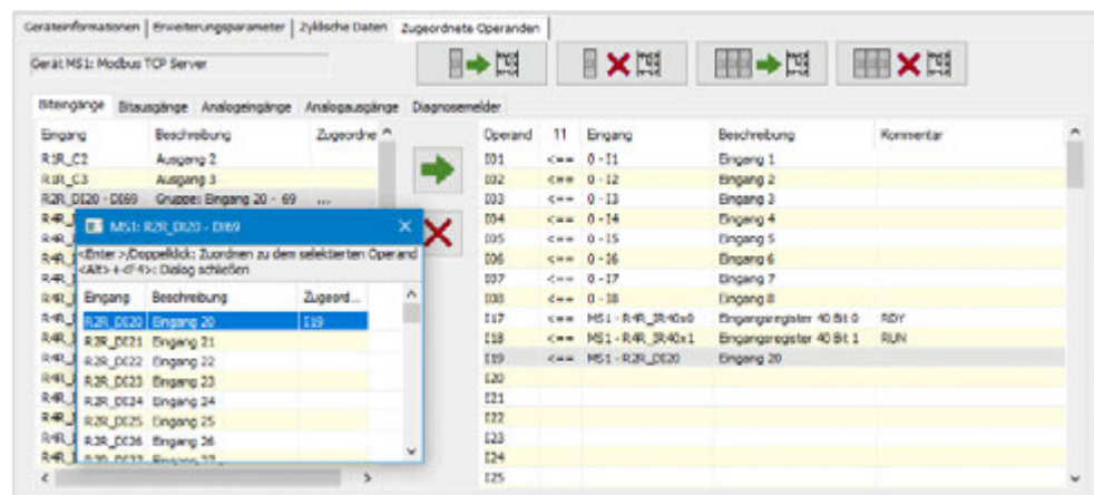
Abb. 391: Register Zugeordnete Operanden Biteingang R2R_DI20 wurde dem Operanden des Basisgerätes 119 bereits zugeordnet.
