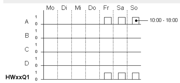
Abb. 126: Wirkdiagramm
