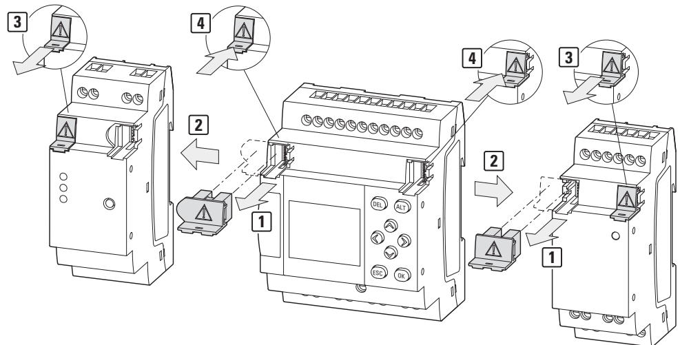
Abb. 15: benachbarte Verbindungsstecker entfernen
