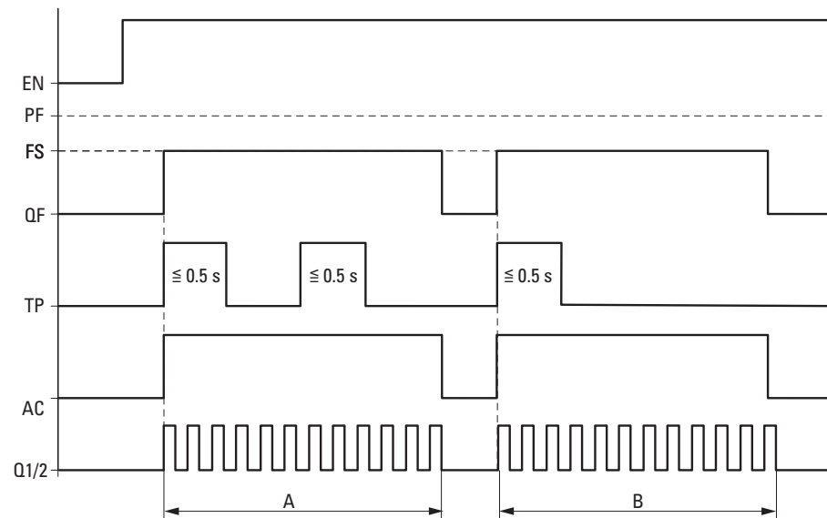
Abb. 200: Wirkdiagramm Tipbetrieb mit vorgegebener Schrittzahl P1
