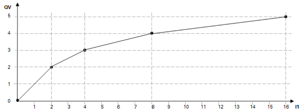
Abb. 188: Beispiel Kennlinie für Funktionsbaustein PM
