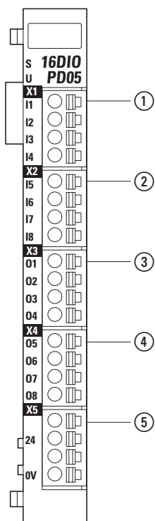
Abbildung 75: Anschlussbelegung
