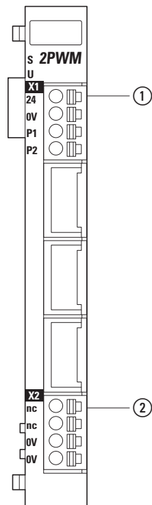
Abbildung 170:Anschlussbelegung
