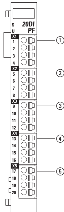
Abbildung 35: Anschlussbelegung
