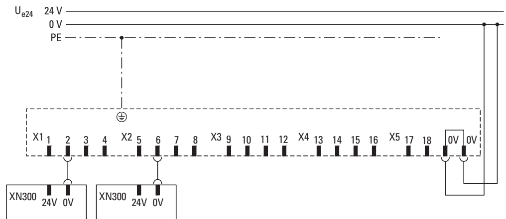
Abbildung 20: Verdrahtungsbeispiel
