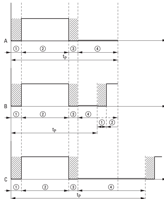
Abbildung 150: Ausgangssignal
