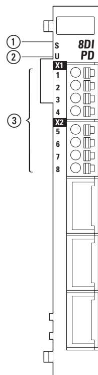
Abbildung 25: Anzeigen und Anschlussbelegung XN-322-8DI-PD
