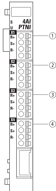
Abbildung 89: Anschlussbelegung
