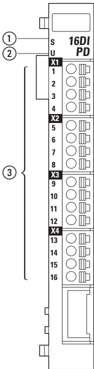
Abbildung 28: Anzeigen und Anschlussbelegung XN-322-16DI-PD 1 Anzeige Status Modul 2 Anzeige User 3 Anzeigen Status der Eingänge 1 bis 16
