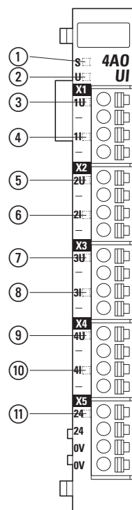
Abbildung 108:Anzeigen
