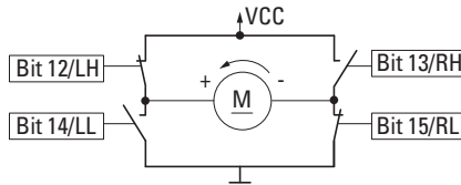
Abbildung 145:Prinzipschaltbild Motordrehrichtung links
