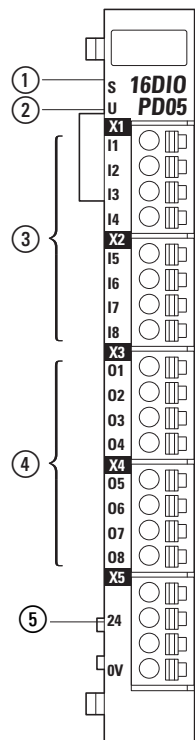
Abbildung 74: Anzeigen XN-322-16DIO-PD05
