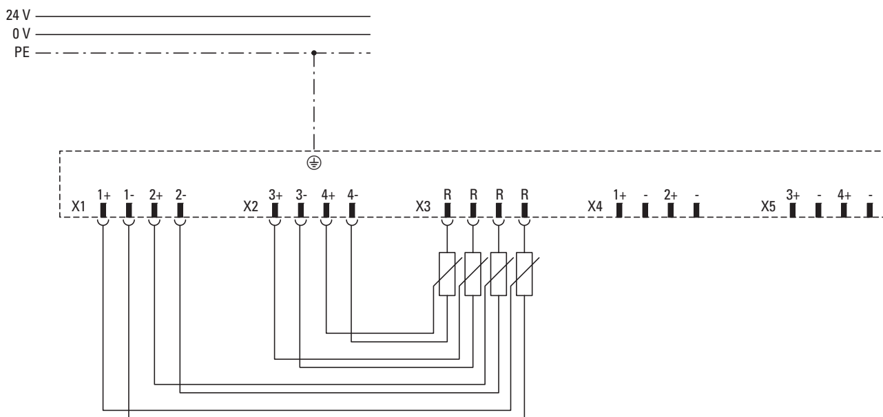
Abbildung 125:Verdrahtung Potentiometermessung
