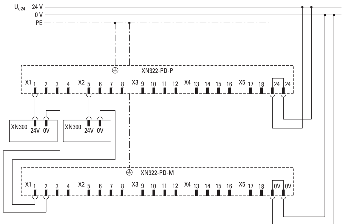
Abbildung 21: Verdrahtungsbeispiel XN-322-18PD-M und XN-322-18PD-P zur Spannungsversorgung von Scheibenmodulen
