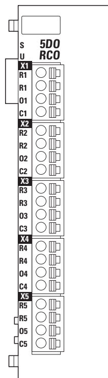
Abbildung 51: Geräteansicht XN-322-5DO-RCO
