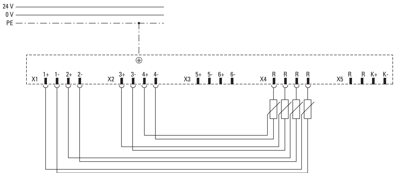
Abbildung 95: Potentiometermessung an AI1, AI2, AI3 und/oder AI4
