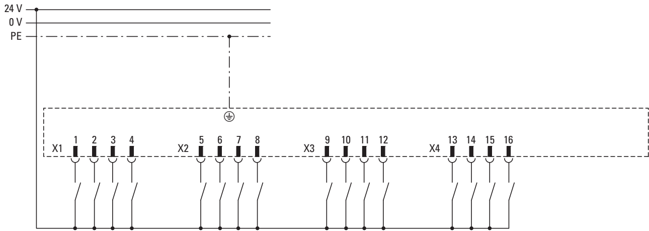
Abbildung 30: Verdrahtung der Eingänge
