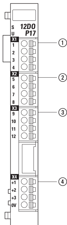
Abbildung 63: Anschlussbelegung
