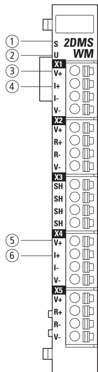
Abbildung 136:Anzeigen und Anschlussbelegung
