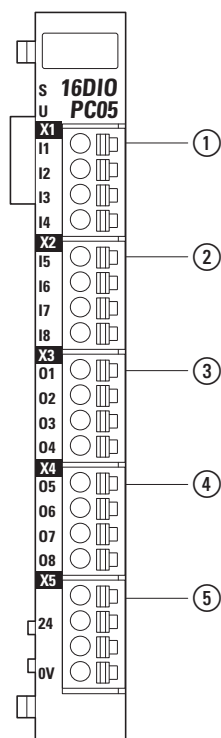
Abbildung 80: Anschlussbelegung
