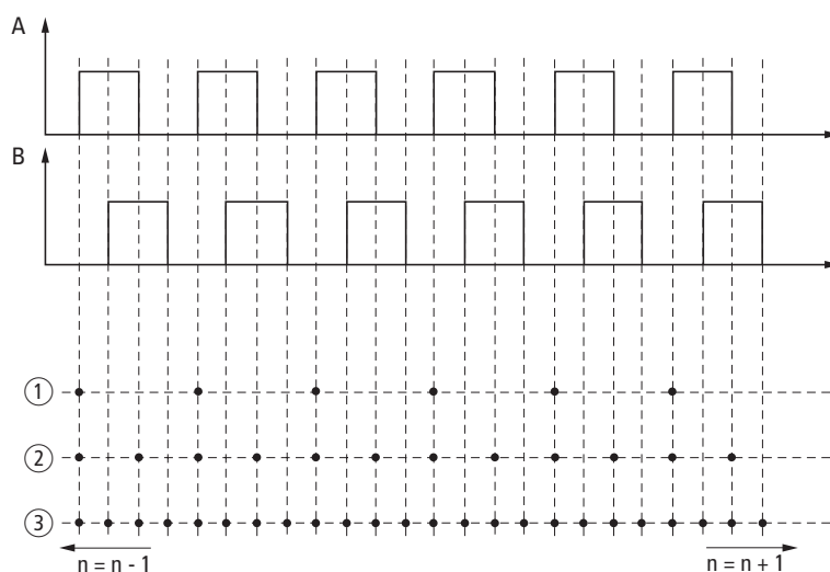
Abbildung 161: Wirkdiagramm Zählermodul
