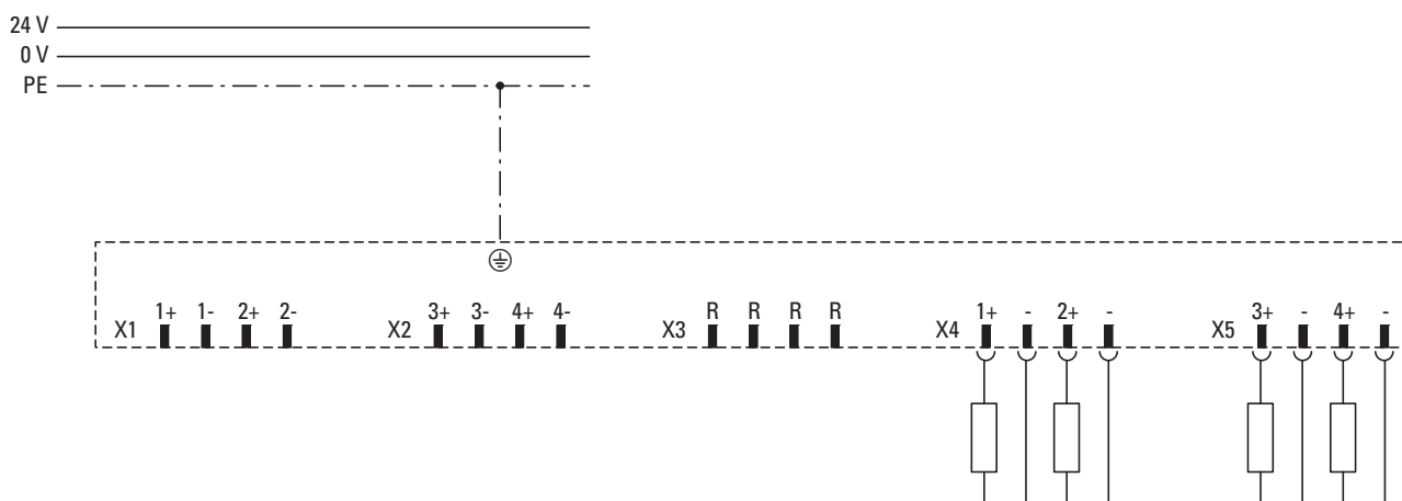
Abbildung 124:Anschluss Analog-Ausgänge
