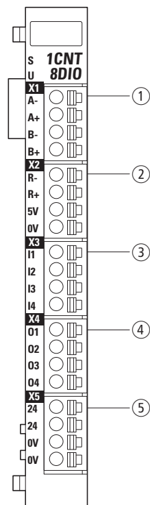
Abbildung 157:Anschlussbelegung
