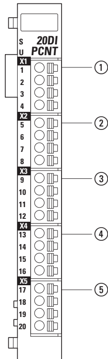
Abbildung 39: Anschlussbelegung
