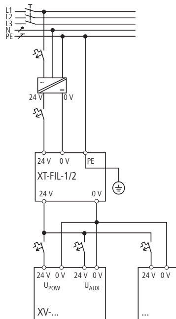
Abbildung 13: Projektierungsbeispiel zur Integration der Entstörfilter
