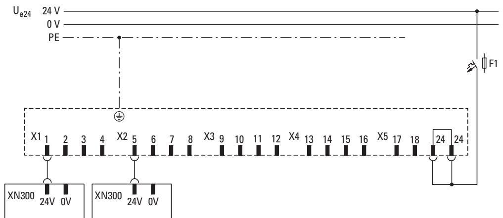
Abbildung 23: Verdrahtungsbeispiel
