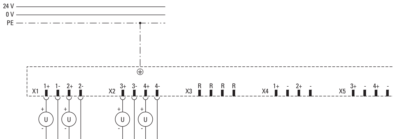
Abbildung 126: Verdrahtung Analog-Eingänge zur Messung eines Gebers
