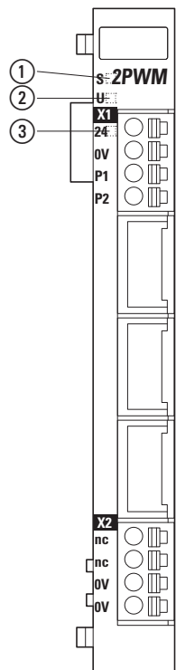
Abbildung 169:Anzeigen und Anschlussbelegung
