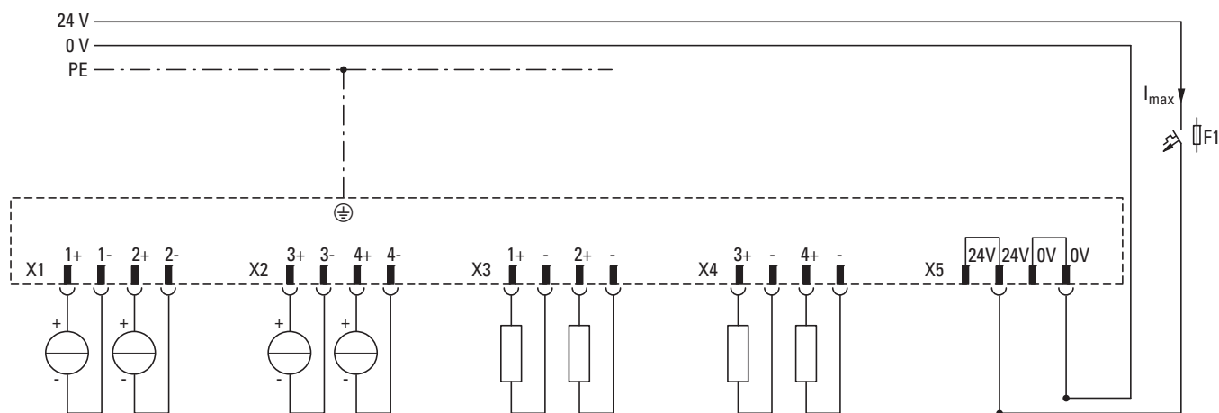
Abbildung 134: Anschlussbeispiel Signal-Stromquellen an X1, X2 und der Bürde-Stromquellen an X3, X4
