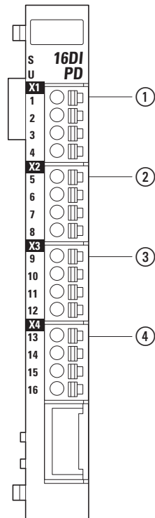
Abbildung 29: Anschlussbelegung
