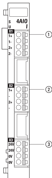
Abbildung 129:Anschlussbelegung
