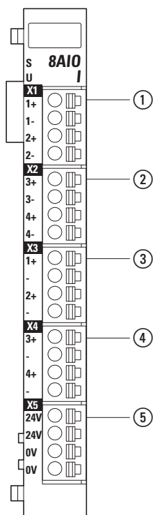
Abbildung 133:Anschlussbelegung
