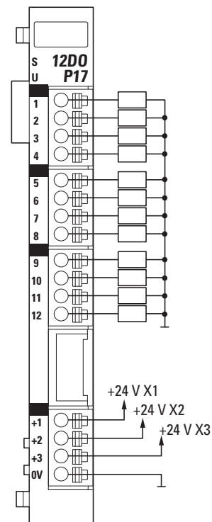
Abbildung 64: Verdrahtungsbeispiel
