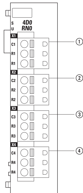
Abbildung 47: Anschlussbelegung
