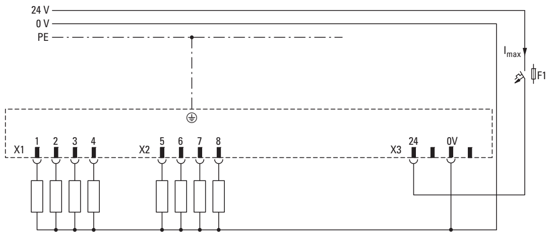
Abbildung 59: Verdrahtungsbeispiel
