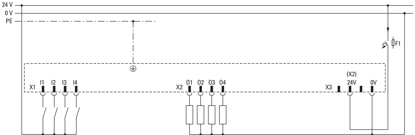
Abbildung 72: Verdrahtung der Eingänge an X1 und der Ausgänge an X2
