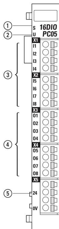
Abbildung 79: Anzeigen XN-322-16DIO-PC05
