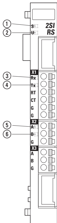
Abbildung 174:Anzeigen 1 Anzeige Status Modul 2 Anzeige User 3 Anzeige RS232 Rx D1 lesen 4 Anzeige RS232 Tx D1 übertragen 5 Anzeige RS485 Rx lesen 6 Anzeige RS485 Tx übertragen
