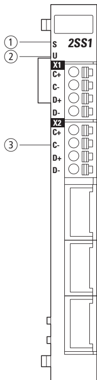
Abbildung 163:Anzeigen XN-322-2SSI
