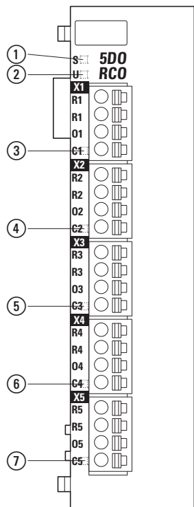
Abbildung 52: Anzeigenbelegung
