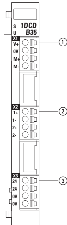
Abbildung 141:Anschlussbelegung XN-322-1DCD-B35
