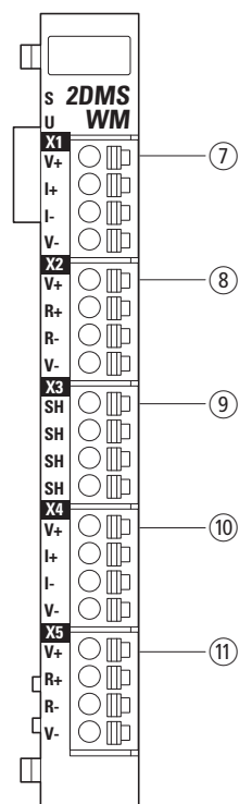
Abbildung 137:Anschlussbelegung
