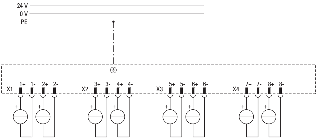
Abbildung 100:Anschlussbeispiel Signal-Stromquellen
