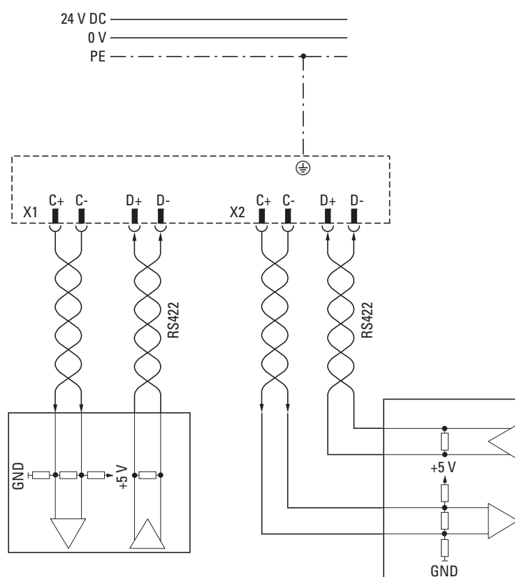
Abbildung 167: Verdrahtungsbeispiel XN-322-2SSI
