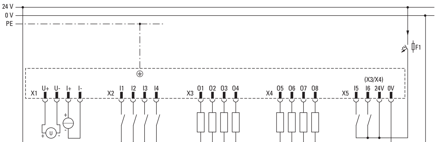
Abbildung 86: Verdrahtung der Eingänge und Ausgänge
