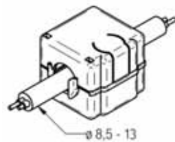
Abbildung 14: Abschirmen mit Einrastferrithülse
