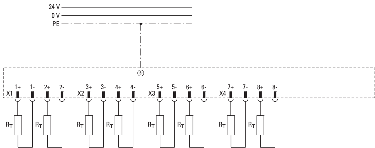
Abbildung 103:Verdrahtungsplan in 2-Leiter-Anschlussstechnik für 8 analoge Eingänge
