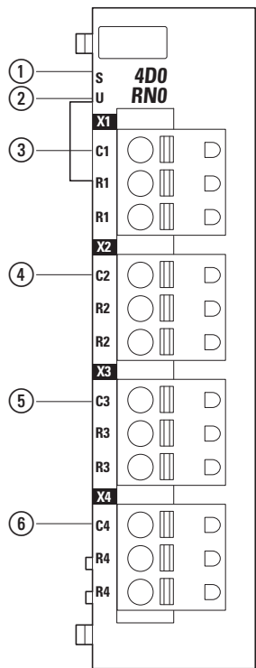
Abbildung 46: Anzeigen und Anschlussbelegung
