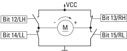
Abbildung 144:Prinzipschaltbild Motordrehrichtung rechts
