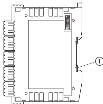
Abbildung 16: Seitansicht XN300 Scheibenmodul
