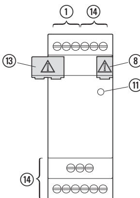
EASY-E4-DC-4PE1(P)
