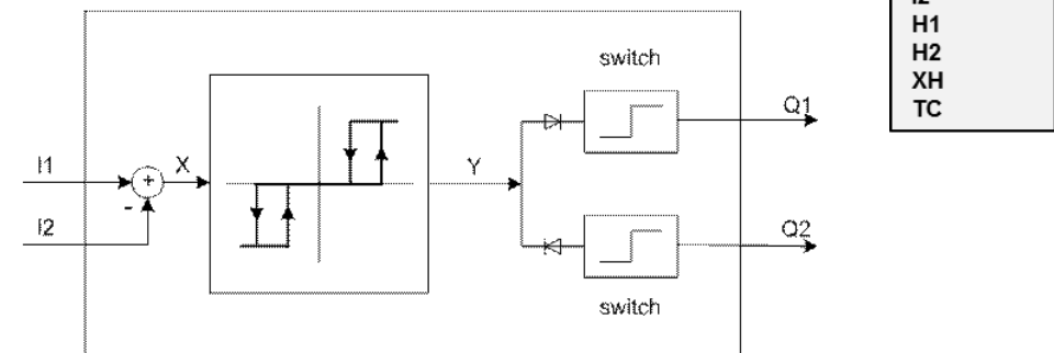
Fig. 203: Schema di principio del regolatore a tre punti
