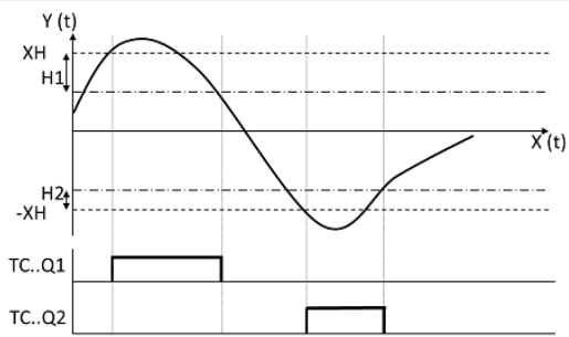
Fig. 205: Diagramma di stato del regolatore a tre punti
