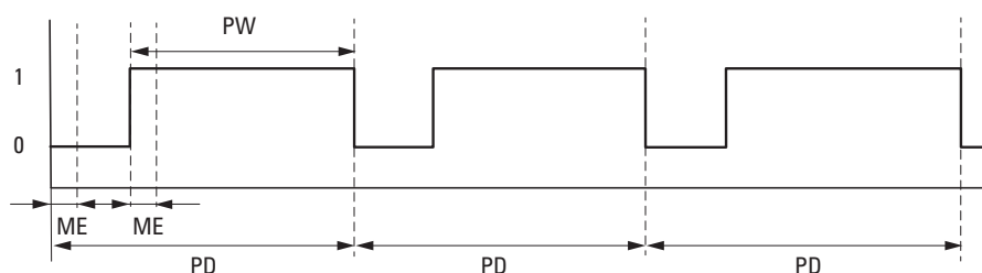
Fig. 190: Impulsions PW sur la sortie du module avec SV = 3218, ME = 93 ms, PD = 1000 ms
