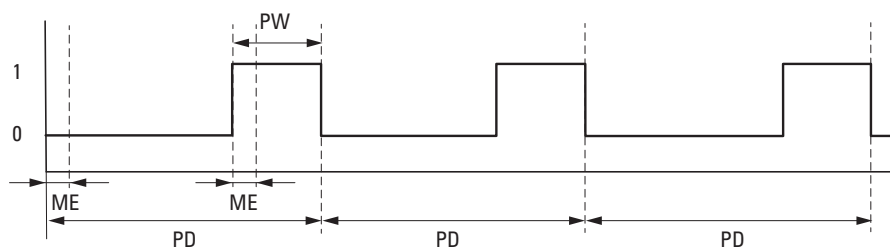
Fig. 189: Impulsions PW sur la sortie du module avec SV = 1400, ME = 93 ms, PD = 1000 ms
