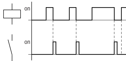
Fig. 103: Diagramme fonctionnel d'une "impulsion sur un cycle" en cas de front descendant
