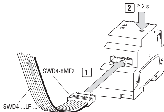
Fig. 346: EASY-COM-SWD-... Raccordement
