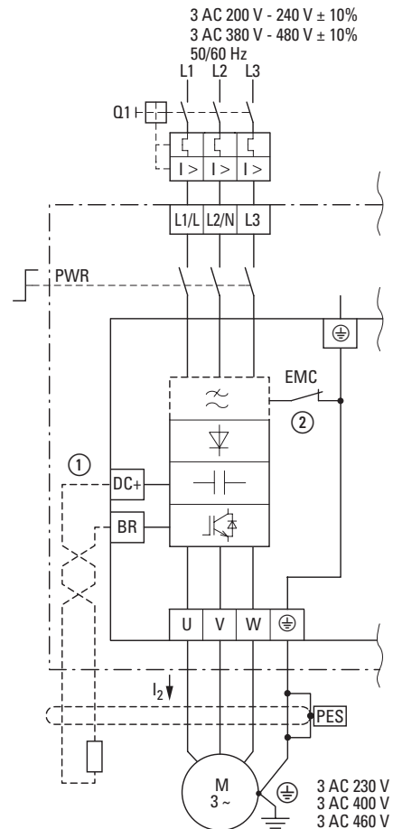
DC1-34...-A6S...
