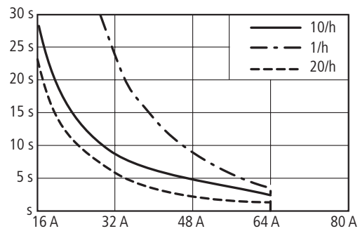
DS7-34x...SX032E...
