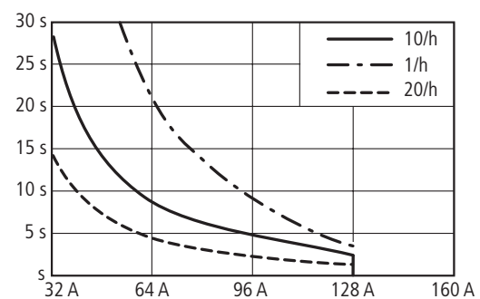
DS7-34x...SX032E...
