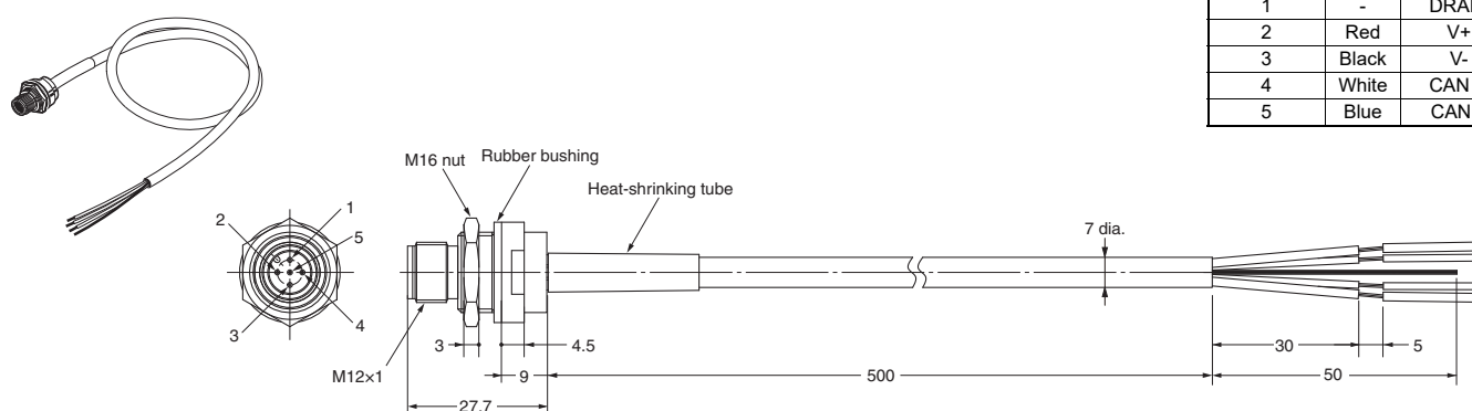
Wiring
