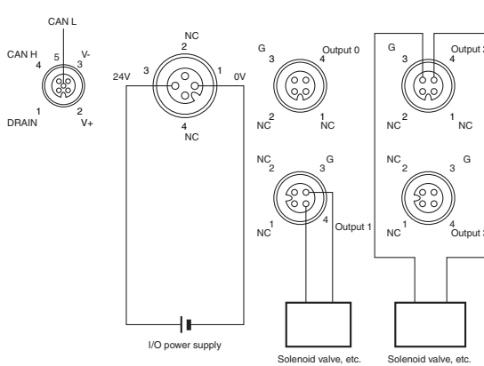
DRT2-OD04CL-1 (PNP)
