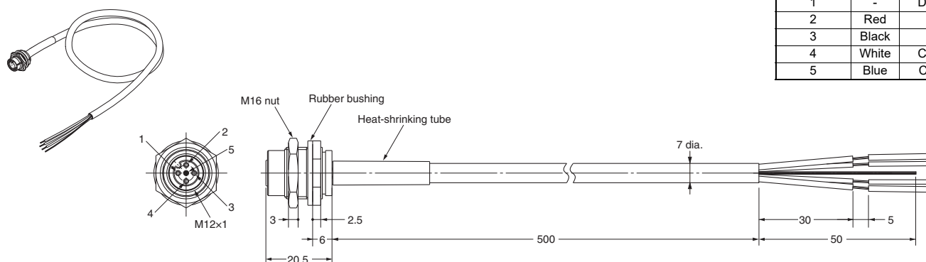
Wiring
