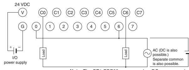
GT1-ROP08/GT1-FOP08
