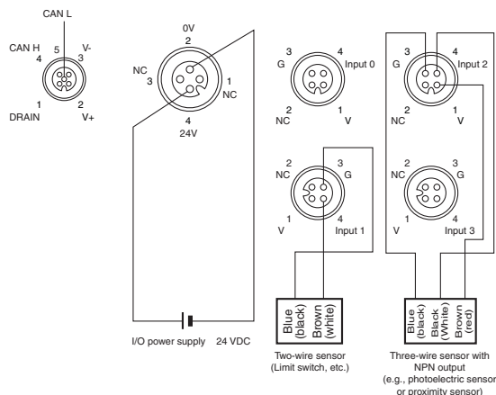
DRT2-OD04CL (NPN)
