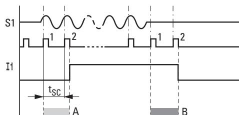
Abb. 310: Schaltverhalten AC-Eingangssignal bei aktivierter I-Entprellung
