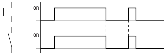
Abb. 97: Wirkdiagramm „Schützfunktion“
