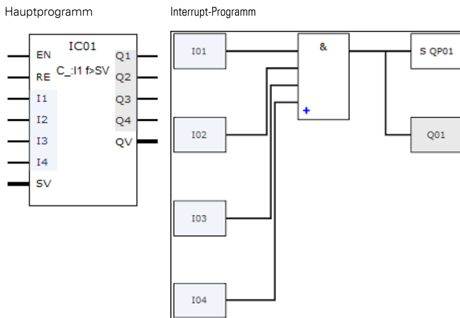
Abb. 257: Übergabe der Zustände von Ein- und Ausgängen zwischen Hauptprogramm und Interrupt-Programm
