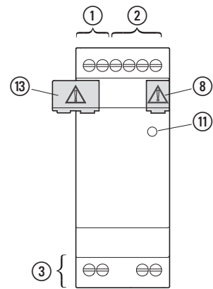
EASY-E4-DC-8TE1(P)
