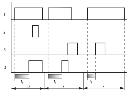
Abb. 146: Wirkdiagramm Zeitrelais ansprechverzögert (mit/ohne Zufallsschalten)
