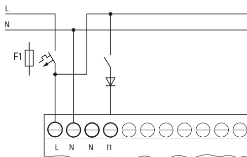
Abb. 4: AC-Eingang mit Entstörsdiode easyE4-AC
