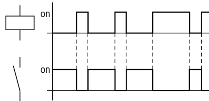
Abb. 101: Wirkdiagramm „inverse Schützfunktion“
