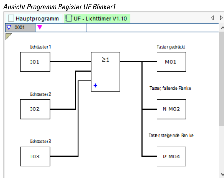
Abb. 276: Ansicht Programm Anwenderbaustein UF Blinker1
