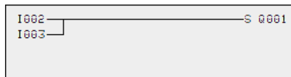
Abb. 116: Parallelschaltung
