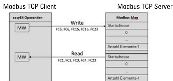
Abb. 239: Übersicht Anwendung der Funktionscodes
