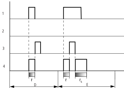
Abb. 151: Wirkdiagramm Zeitrelais, Impulsformend 2
