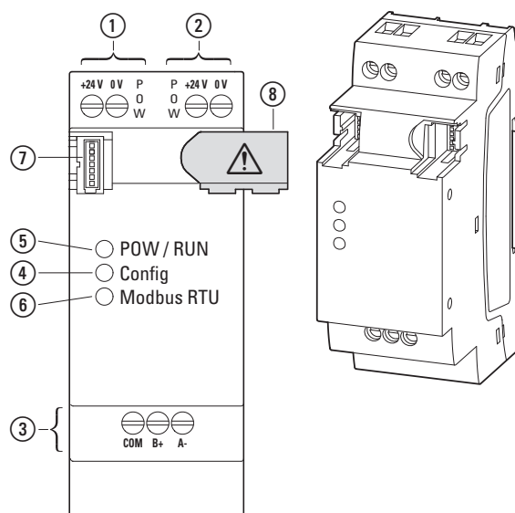
Abb. 349: Geräteübersicht
