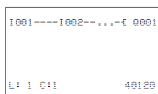
Abb. 84: Schaltplan mit Eingängen I01, I02 und Ausgang Q1
