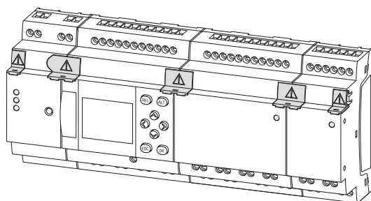
Abb. 343: Beispiel Steuerrelais easyE4 mit E/A-Erweiterungen und easy Kommunikationsmodul EASY-COM-SWD-...
