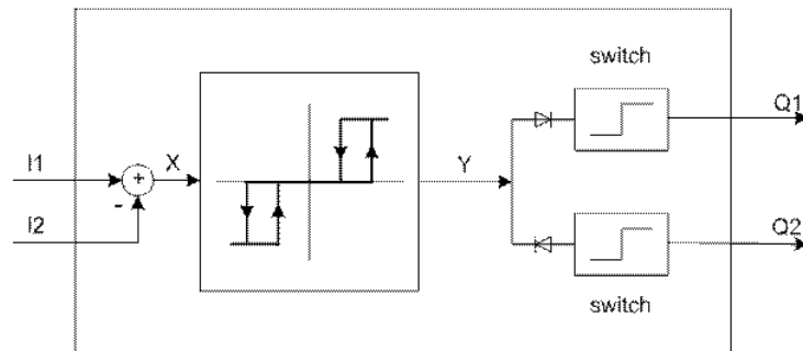
Abb. 203: Prinzipschaltbild Dreipunktregler
