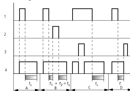
Abb. 147: Wirkdiagramm Zeitrelais rückfallverzögert (mit/ohne Zufallsschalten, mit/ohne Retriggerung)
