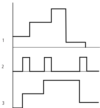
Abb. 214: Wirkdiagramm Datenbaustein
