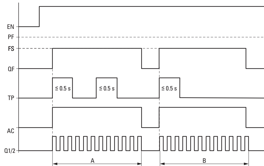
Abb. 200: Wirkdiagramm Tippbetrieb mit vorgegebener Schrittzahl P1
