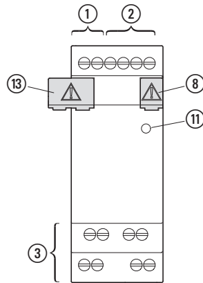
EASY-E4-...-8...
