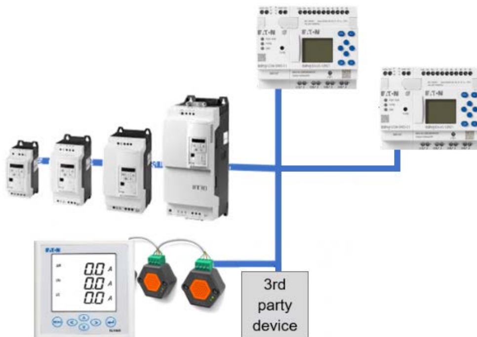
Abb. 348: Übersicht: easyE4 als Modbus RTU Master kommuniziert mit DE1, DC1, DG1, DA1, easyE4 als Modbus RTU Slave und anderen Geräten
