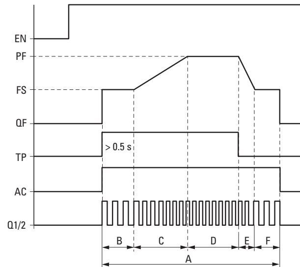
Abb. 202: Wirkdiagramm Tippbetrieb mit vorgegebener Tippfrequenz, P1 nach Bremsphase nicht erreicht
