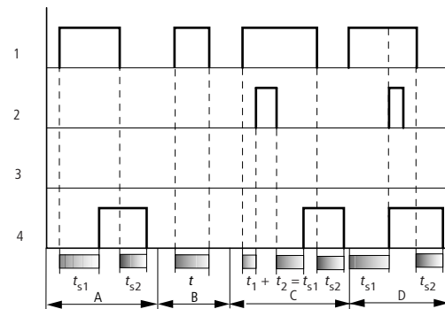
Abb. 149: Wirkdiagramm Zeitrelais, ansprech- und rückfallverzögert
