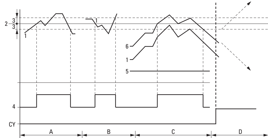
Abb. 178: Wirkdiagramm Analogwerte-Vergleicher
