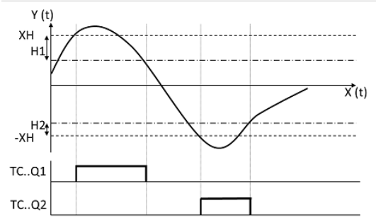
Abb. 205: Wirkdiagramm Dreipunktregler
