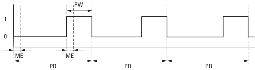
Abb. 189: Impulse PW am Bausteinausgang bei SV =1400, ME = 93 ms, PD=1000 ms
