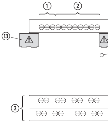
EASY-E4-...-16...
