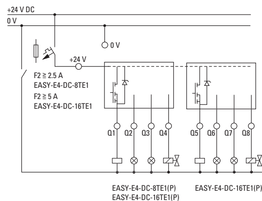
Abb. 25: Transistor-Ausgang Erweiterungsgerät anschließen
