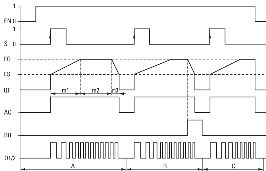
Abb. 199: Wirkdiagramm Impulsausgabe PO bei vorgegebener Impulsanzahl I1 - mögliche Phasen des Normalbetriebs
