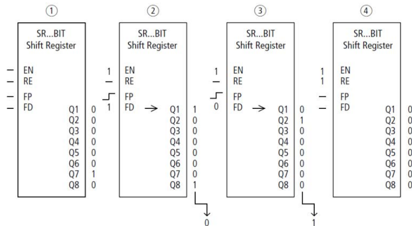
Abb. 219: Schieberegister SR.: Vorwärtsoperation in der Betriebsart BIT
