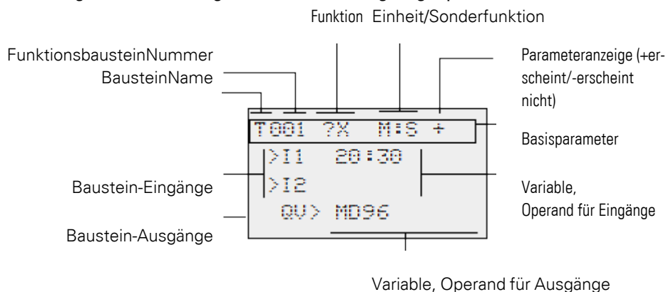
Abb. 121: Anzeige der Herstellerbausteine im Bausteineditor
