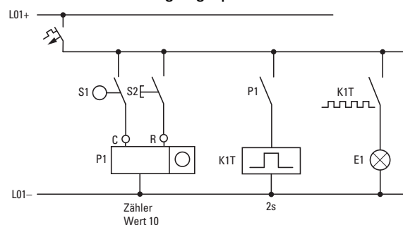
Abb. 290: Festverdrahtung mit Relais
