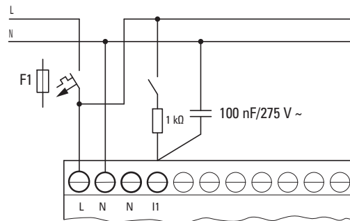
Abb. 7: Begrenzung des Eingangsstromes durch Widerstand
