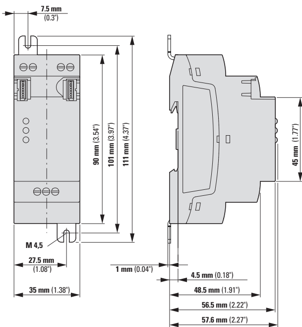
Abb. 403: Abmessungen in mm (Inch) Erweiterungen 2TE
