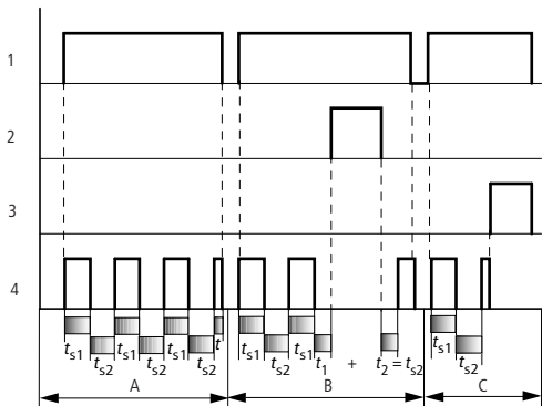
Abb. 152: Wirkdiagramm Zeitrelais, Impulsformend
