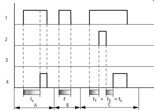
Abb. 145: Wirkdiagramm Zeitrelais ansprechverzögert (mit/ohne Zufallsschalten)
