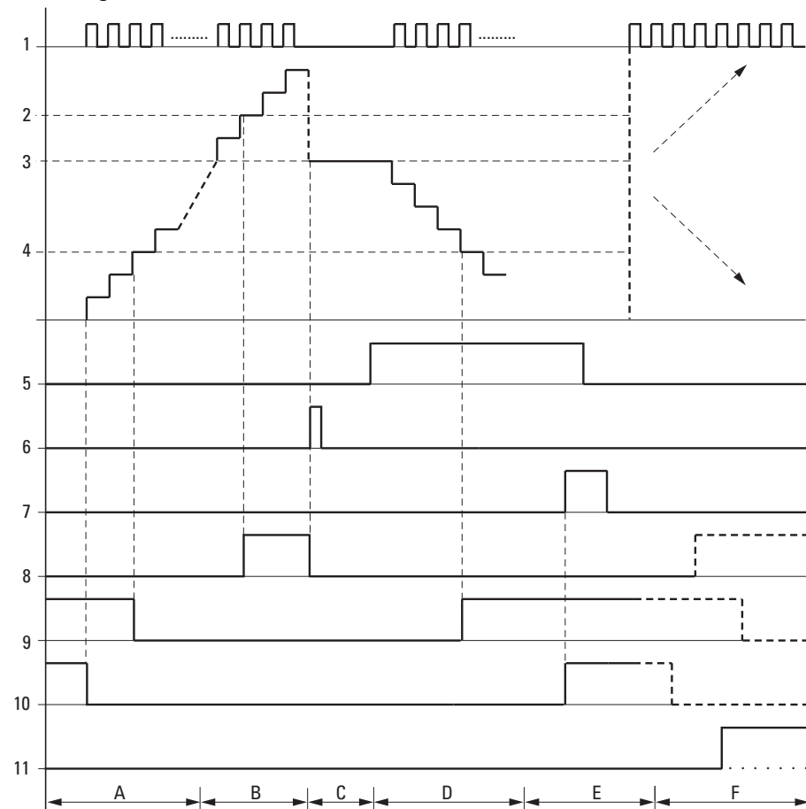
Abb. 172: Wirkdiagramm Zählrelais
