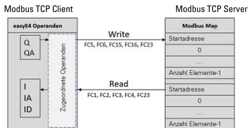
Abb. 389: Überblick Funktionscodes Zyklische Daten
