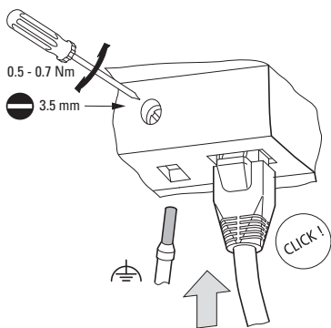
Abb. 37: Ethernet-Leitung anschließen
