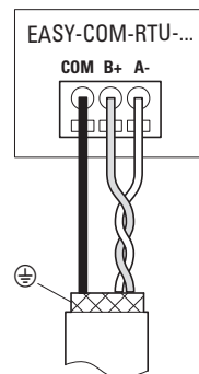
Abb. 350: EASY-COM-RTU-... Ausgänge anschließen
