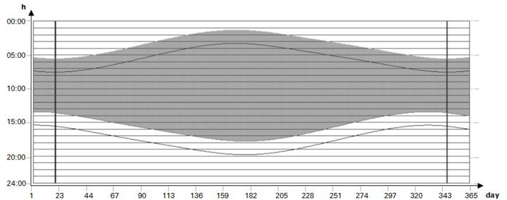
Abb. 169: Offset; O1=-2; O2=-2; Q1=1 schaltet 2 Stunden vor Sonnenaufgang ein und 2 Stunden vor Sonnenuntergang aus
