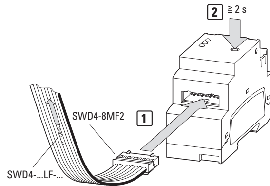
Abb. 346: EASY-COM-SWD-... anschließen
