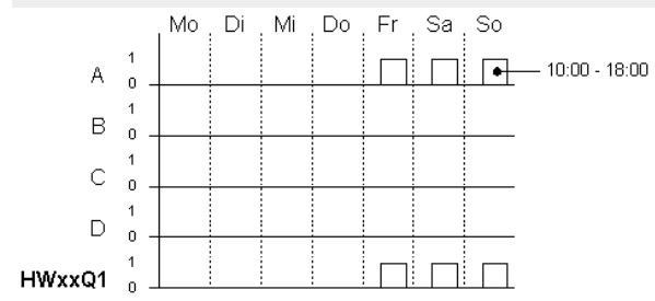
Abb. 126: Wirkdiagramm
