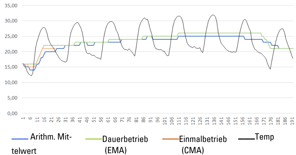
Abb. 182: Beispielkennlinie Temperaturmessung stündlich, über 7 Tage
