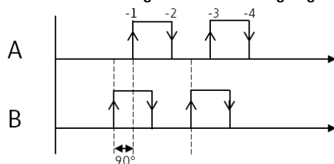
Abb. 176: Funktionsbaustein CI rückwärts zählend; QV=QV-4
