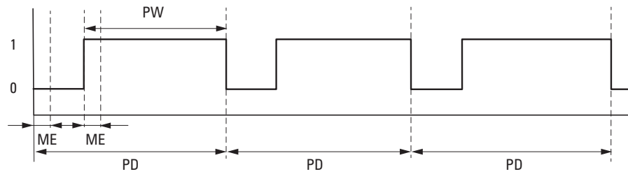
Abb. 190: Impulse PW am Bausteinausgang bei SV = 3218, ME = 93 ms, PD=1000 ms
