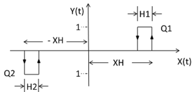
Abb. 204: Zeitdiagramm Dreipunktregler
