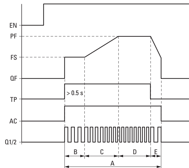
Abb. 201: Wirkdiagramm Tipbetrieb mit vorgegebener Tippfrequenz, P1 nach Bremsphase erreicht
