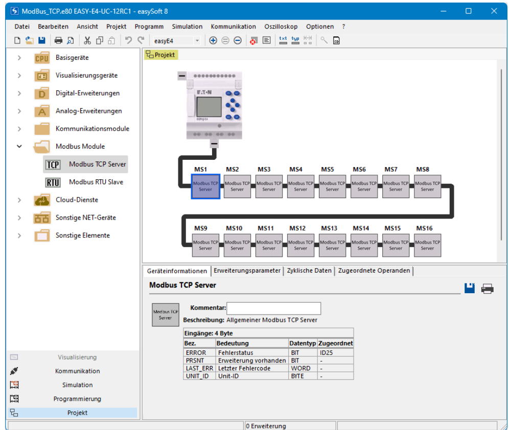
Abb. 384: Arbeitsfläche mit Basisgerät und Modbus TCP Server Module
