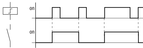
Abb. 98: Wirkdiagramm „Stromstoßrelais“
