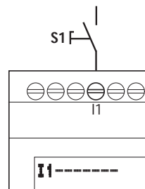
Abb. 306: easyE4-Eingang mit Schalter belegt
