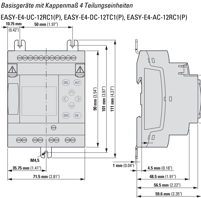
Abb. 397: Abmessungen in mm (Inch) Basisgeräte EASY-E4-...-12...C1(P)
