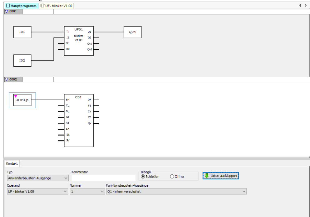
Abb. 279: Ein-/Ausgänge verdrahten
