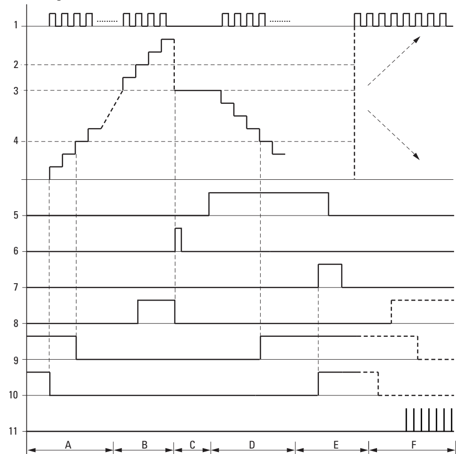
Abb. 177: Wirkdiagramm Schneller Inkrementalwertzähler
