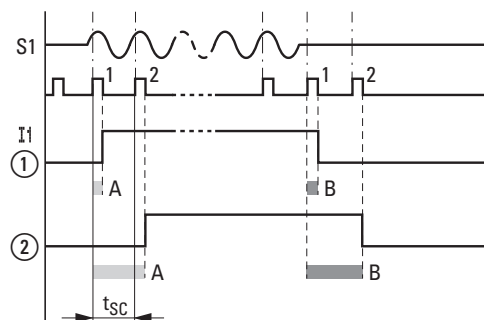
Abb. 309: Verzögerungszeiten bei der Auswertung eines AC-Eingangssignales
