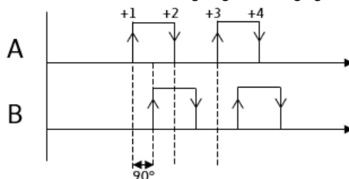
Abb. 175: Funktionsbaustein CI vorwärts zählend; QV=QV+4
