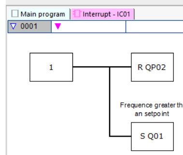
Abb. 265: easySoft 8 Interrupt-Programm Frequenzmessung
