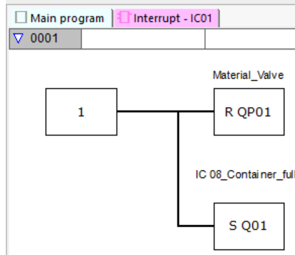
Abb. 261: easySoft 8 Interrupt-Programm zwei Zählereingänge
