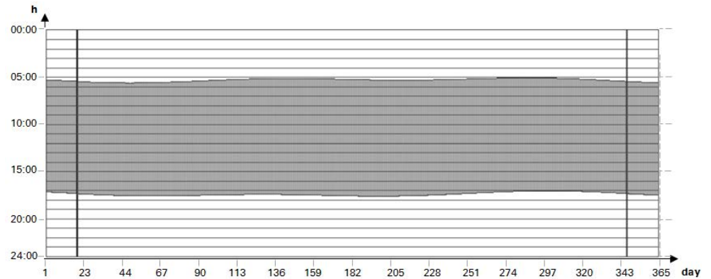
Abb. 165: Offset; O1=-2; O2=2; Q1=1 schaltet 2 Stunden vor Sonnenaufgang ein und 2 Stunden nach Sonnenuntergang aus
