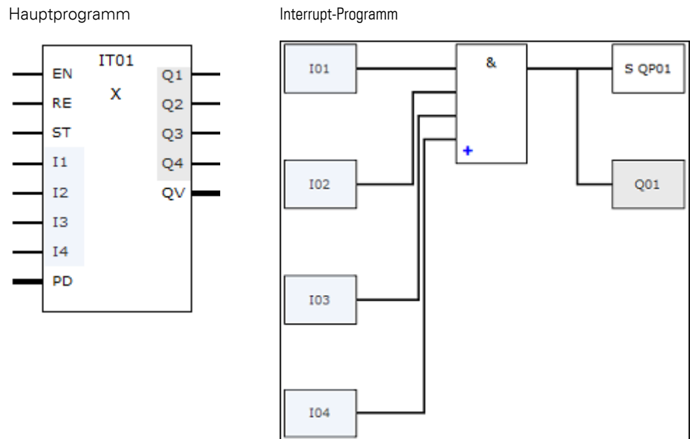
Abb. 269: Übergabe der Zustände von Ein- und Ausgängen zwischen Hauptprogramm und Interrupt-Programm
