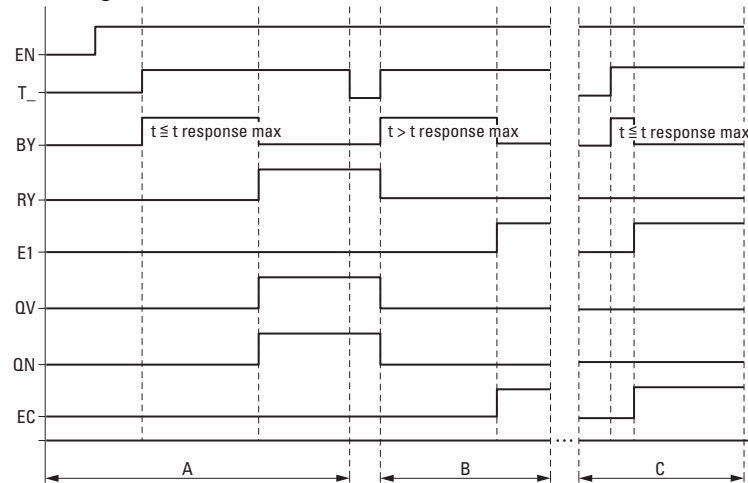
Abb. 252: Wirkdiagramm Frequenzzähler
