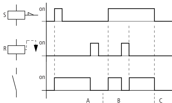
Abb. 99: Wirkdiagramm „Setzen“ und „Rücksetzen“
