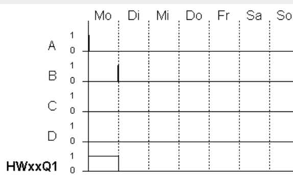
Abb. 134: Wirkdiagramm
