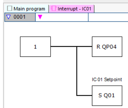
Abb. 259: easySoft 8 Interrupt-Programm Impulszähler mit externer Richtung
