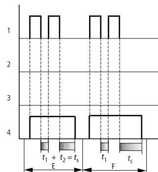
Abb. 148: Wirkdiagramm Zeitrelais rückfallverzögert (mit/ohne Zufallsschalten, mit/ohne Retriggerung)
