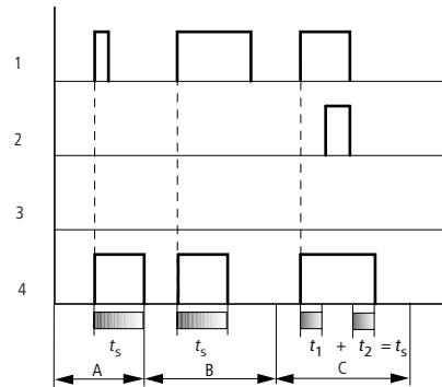
Abb. 150: Wirkdiagramm Zeitrelais, Impulsformend 1
