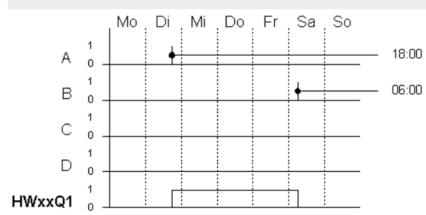
Abb. 130: Wirkdiagramm
