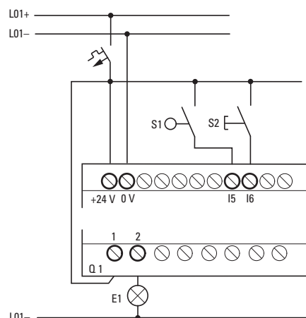
Abb. 291: Verdrahtung z.B. mit EASY-E4-UC-...
