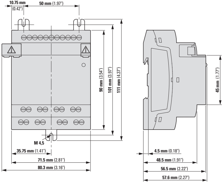
Abb. 399: Abmessungen in mm (Inch) Erweiterungen 4TE
