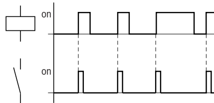
Abb. 102: Wirkdiagramm „Zyklusimpuls“ bei positiver Flanke
