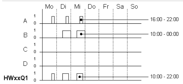
Abb. 132: Wirkdiagramm
