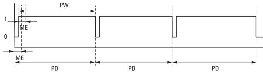
Abb. 191: Am Bausteinausgang wird Dauersignal angezeigt bei SV = 3768, ME = 93 ms, PD=1000 ms; E1 = 1
