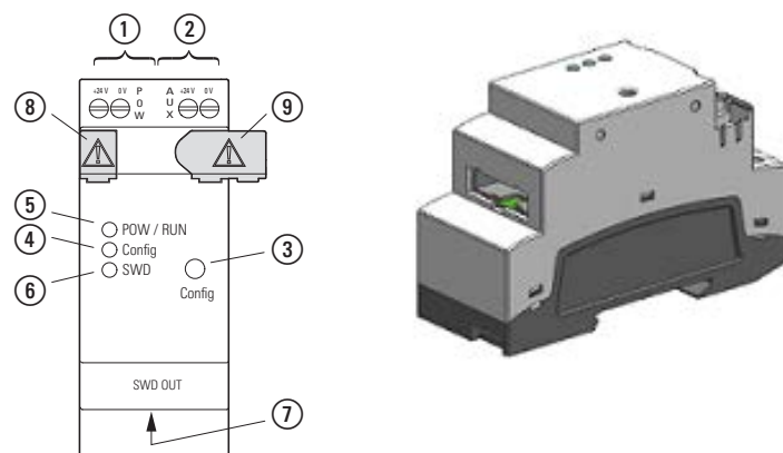
Abb. 344: Geräteausführung in 2TE
