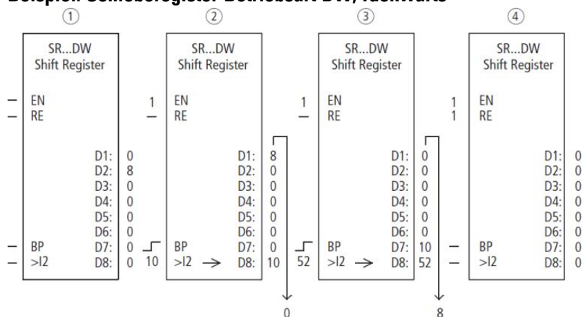
Abb. 220: Schieberegister SR.: Rückwärtsoperation in der Betriebsart DW
