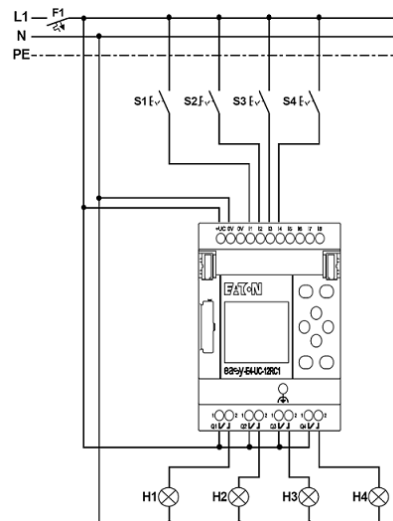
Abb. 405: Schaltplan easyE4 Lauflicht
