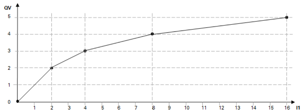
Abb. 188: Beispiel Kennlinie für Funktionsbaustein PM
