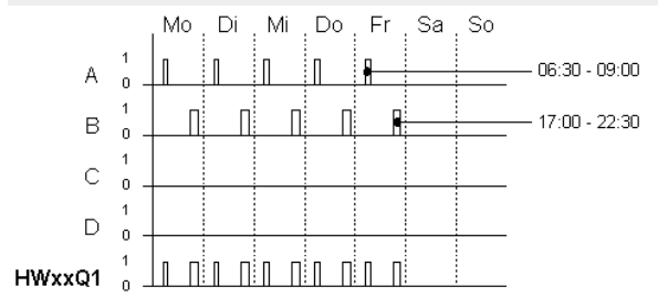
Abb. 128: Wirkdiagramm
